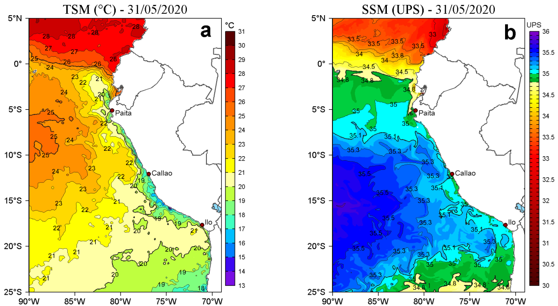
Figura 2. a) Temperatura superficial del mar (TSM, °C) y b) Salinidad superficial del mar (SSM, UPS), para el 31 de mayo de 2020. Datos: OSTIA-UKMO-L4-GLOB-v2.0 (UK Met Office, 2012; Donlon et al, 2012) disponible en https://podaac.jpl.nasa.gov/dataset/OSTIA-UKMO-L4-GLOB-v2.0 para (a) y Hybrid Coordinate Ocean Model v. GOFS 3.1 (HYCOM; Halliwell et al., 1998; 2000; Bleck, 2001) para (b). Procesamiento: LHFM/AFIOF/DGIOCC/IMARPE.
