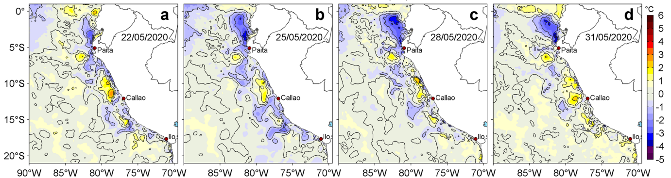
Figura 3. Anomalías de la temperatura superficial del mar (TSM, °C) para los días: a) 22, b) 25, c) 28 y d) 31 de mayo de 2020. Las anomalías se calcularon respecto de la climatología para el periodo 2007-2016. Datos: OSTIA-UKMO-L4-GLOB-v2.0 (UK Met Office, 2012; Donlon et al, 2012). Procesamiento: LHFM/AFIOF/DGIOCC/IMARPE.
