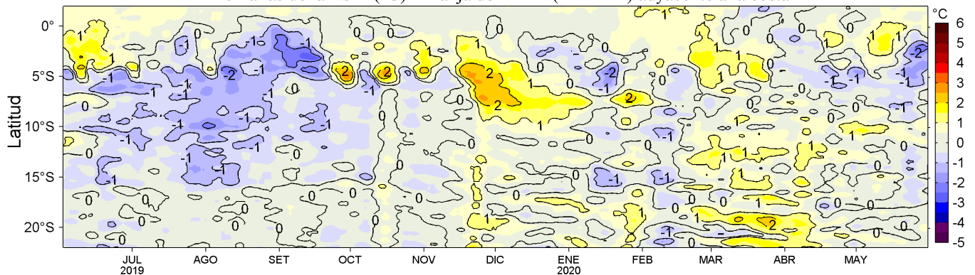
Figura 4. Variación promedio de las anomalías de la temperatura superficial del mar (TSM, °C) para una franja de 60 mn (~111 km) adyacente al litoral peruano para los últimos doce meses al 31 de mayo de 2020. Datos: OSTIA-UKMO-L4-GLOB-v2.0 (UK Met. Office, 2012; Donlon et al, 2012) disponible en https://podaac.jpl.nasa.gov/dataset/OSTIA-UKMO-L4-GLOB-v2.0 . Las anomalías se calcularon con respecto al periodo 2007-2016. Procesamiento: LHFM/AFIOF/DGIOCC/IMARPE.
