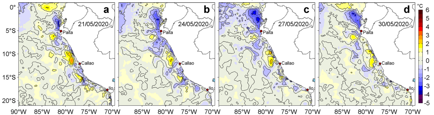
Figura 3. Anomalías de la temperatura superficial del mar (TSM, °C) para los días: a) 21, b) 24, c) 27 y d) 30 de mayo de 2020. Las anomalías se calcularon respecto de la climatología para el periodo 2007-2016. Datos: OSTIA-UKMO-L4-GLOB-v2.0 (UK Met Office, 2012; Donlon et al, 2012). Procesamiento: LHF/M/AFIOF/DGIOCC/IMARPE.
