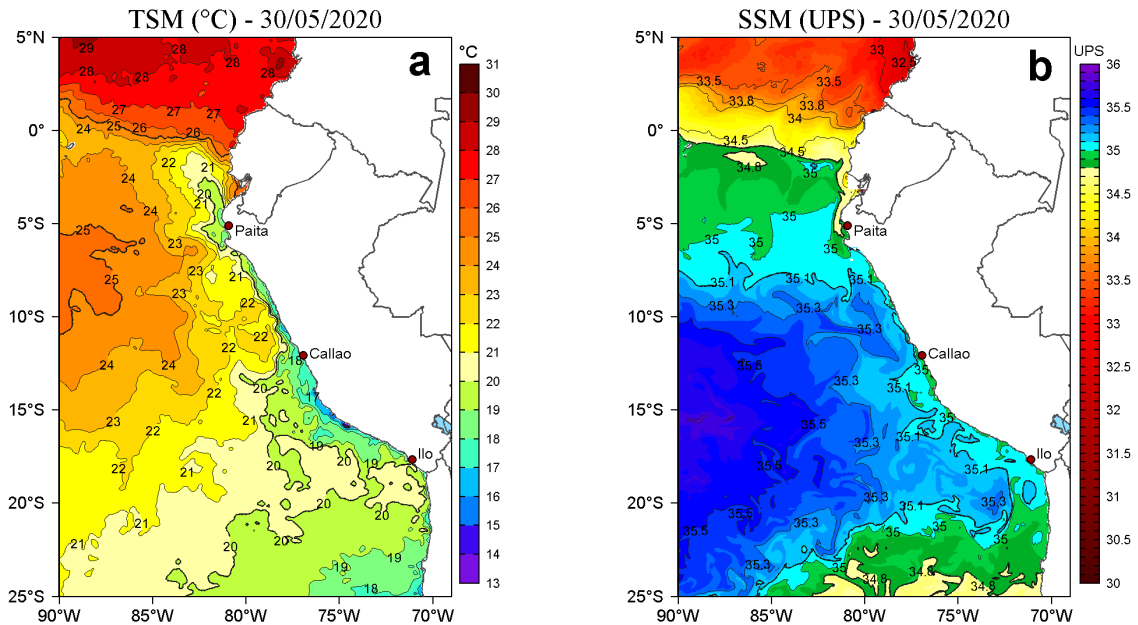
Figura 2. a) Temperatura superficial del mar (TSM, °C) y b) Salinidad superficial del mar (SSM, UPS), para el 30 de mayo de 2020. Datos: OSTIA-UKMO-L4-GLOB-v2.0 (UK Met Office, 2012; Donlon et al, 2012) disponible en https://podaac.jpl.nasa.gov/dataset/OSTIA-UKMO-L4-GLOB-v2.0 para (a) y Hybrid Coordinate Ocean Model v. GOFS 3.1 (HYCOM; Halliwell et al., 1998; 2000; Bleck, 2001) para (b). Procesamiento: LHF/M/AFIOF/DGIOCC/IMARPE.
