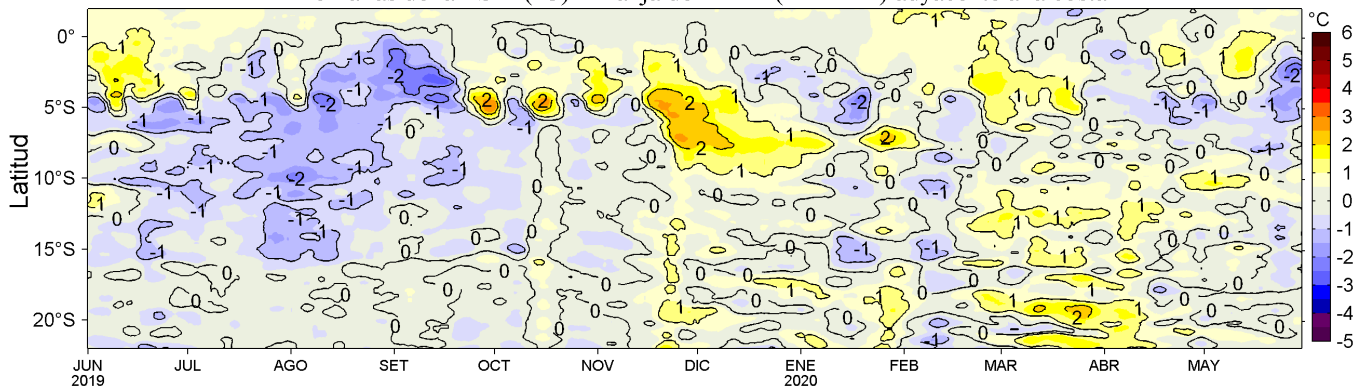
Figura 4. Variación promedio de las anomalías de la temperatura superficial del mar (TSM, °C) para una franja de 60 mn (~111 km) adyacente al litoral peruano para los últimos doce meses al 30 de mayo de 2020. Datos: OSTIA-UKMO-L4-GLOB-v2.0 (UK Met. Office, 2012; Donlon et al, 2012) disponible en https://podaac.jpl.nasa.gov/dataset/OSTIA-UKMO-L4-GLOB-v2.0 . Las anomalías se calcularon con respecto al periodo 2007-2016. Procesamiento: LHF/M/AFIOF/DGIOCC/IMARPE.
