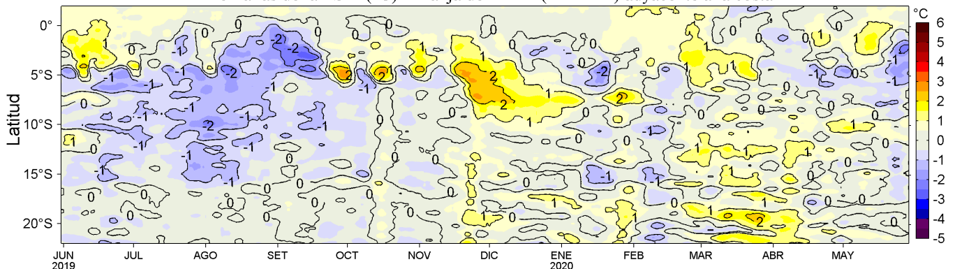
Figura 4. Variación promedio de las anomalías de la temperatura superficial del mar (TSM, °C) para una franja de 60 mn (~111 km) adyacente al litoral peruano para los últimos doce meses al 29 de mayo de 2020. Datos: OSTIA-UKMO-L4-GLOB-v2.0 (UK Met. Office, 2012; Donlon et al, 2012) disponible en https://podaac.jpl.nasa.gov/dataset/OSTIA-UKMO-L4-GLOB-v2.0 . Las anomalías se calcularon con respecto al periodo 2007-2016. Procesamiento: LHFM/AFIOF/DGIOCC/IMARPE.
