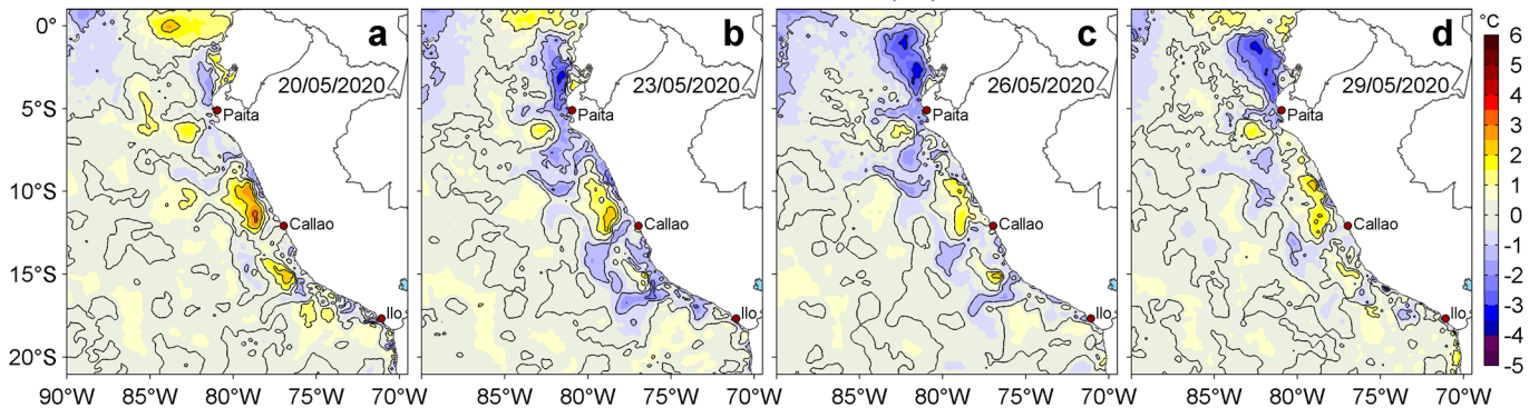
Figura 3. Anomalías de la temperatura superficial del mar (TSM, °C) para los días: a) 20, b) 23, c) 26 y d) 29 de mayo de 2020. Las anomalías se calcularon respecto de la climatología para el periodo 2007-2016. Datos: OSTIA-UKMO-L4-GLOB-v2.0 (UK Met Office, 2012; Donlon et al, 2012). Procesamiento: LHFM/AFIOF/DGIOCC/IMARPE.
