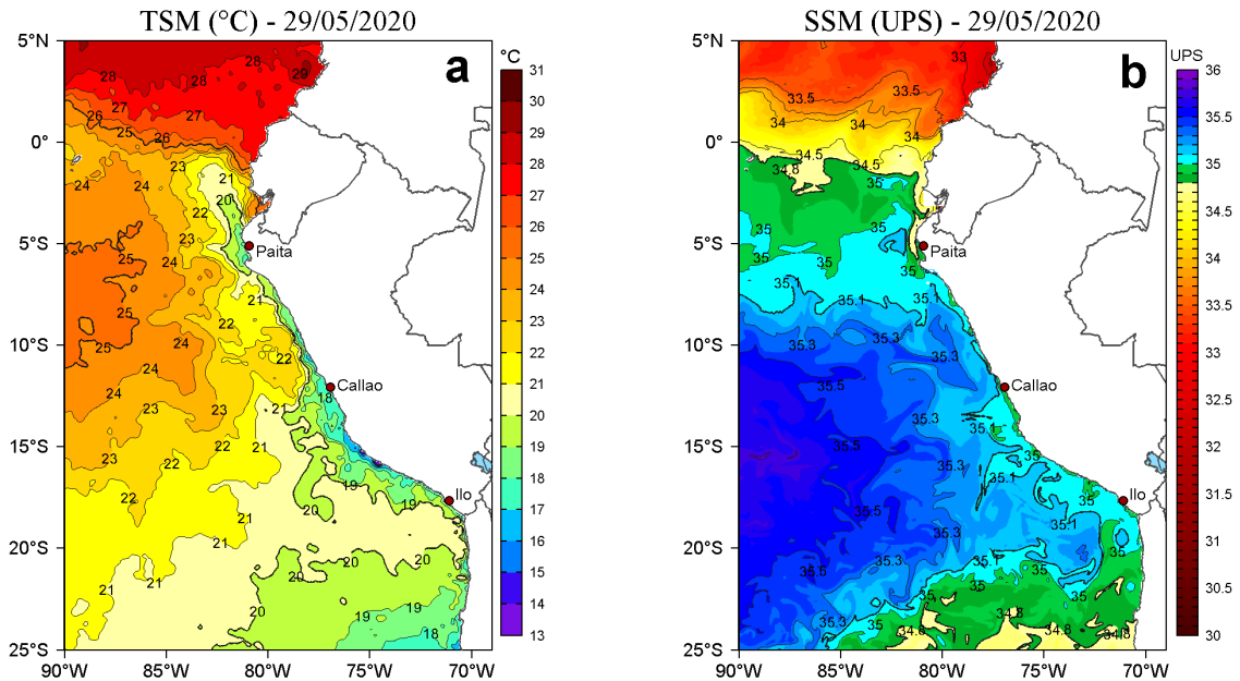
Figura 2. a) Temperatura superficial del mar (TSM, °C) y b) Salinidad superficial del mar (SSM, UPS), para el 29 de mayo de 2020. Datos: OSTIA-UKMO-L4-GLOB-v2.0 (UK Met Office, 2012; Donlon et al, 2012) disponible en https://podaac.jpl.nasa.gov/dataset/OSTIA-UKMO-L4-GLOB-v2.0 para (a) y Hybrid Coordinate Ocean Model v. GOFS 3.1 (HYCOM; Halliwell et al., 1998; 2000; Bleck, 2001) para (b). Procesamiento: LHFM/AFIOF/DGIOCC/IMARPE.
