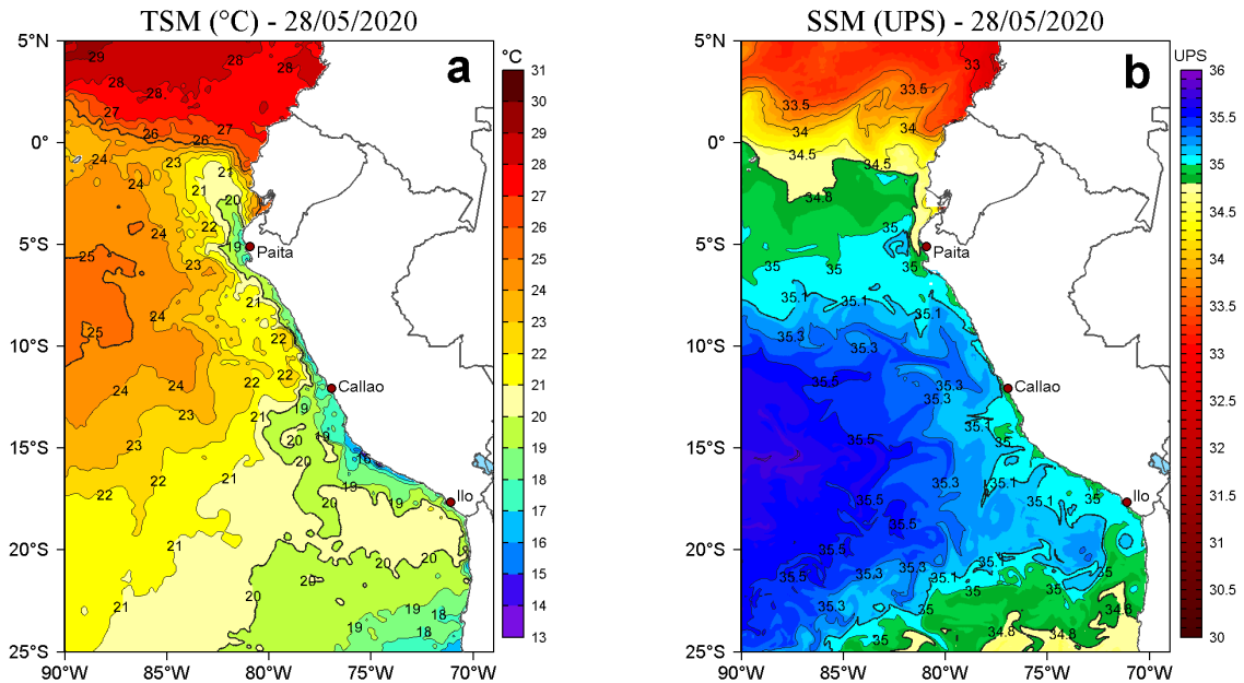
Figura 2. a) Temperatura superficial del mar (TSM, °C) y b) Salinidad superficial del mar (SSM, UPS), para el 28 de mayo de 2020. Datos: OSTIA-UKMO-L4-GLOB-v2.0 (UK Met Office, 2012; Donlon et al, 2012) disponible en https://podaac.jpl.nasa.gov/dataset/OSTIA-UKMO-L4-GLOB-v2.0 para (a) y Hybrid Coordinate Ocean Model v. GOFS 3.1 (HYCOM; Halliwell et al., 1998; 2000; Bleck, 2001) para (b). Procesamiento: LHFM/AFIOF/DGIOCC/IMARPE.
