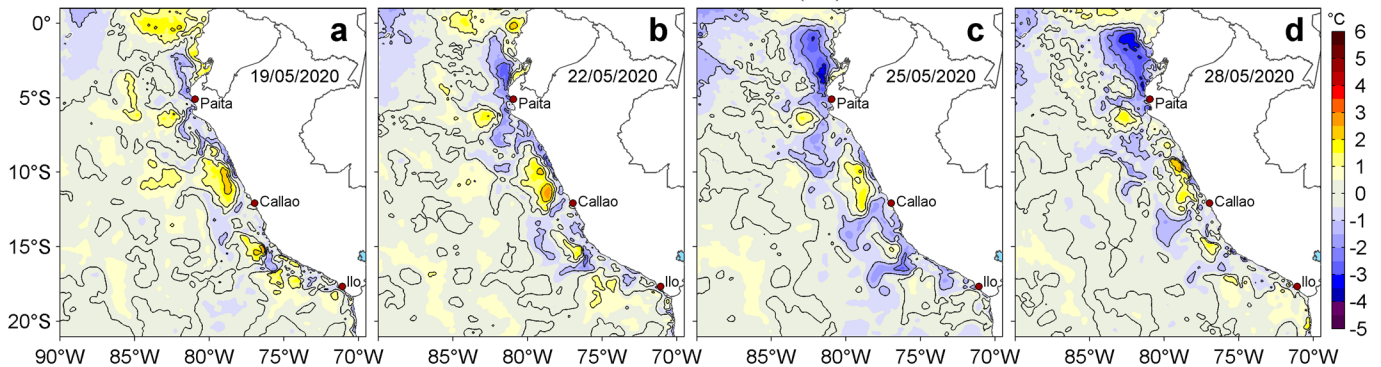
Figura 3. Anomalías de la temperatura superficial del mar (TSM, °C) para los días: a) 19, b) 22, c) 25 y d) 28 de mayo de 2020. Las anomalías se calcularon respecto de la climatología para el periodo 2007-2016. Datos: OSTIA-UKMO-L4-GLOB-v2.0 (UK Met Office, 2012; Donlon et al, 2012). Procesamiento: LHFM/AFIOF/DGIOCC/IMARPE.
