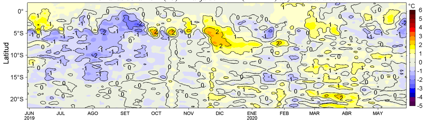
Figura 4. Variación promedio de las anomalías de la temperatura superficial del mar (TSM, °C) para una franja de 60 mn (~111 km) adyacente al litoral peruano para los últimos doce meses al 28 de mayo de 2020. Datos: OSTIA-UKMO-L4-GLOB-v2.0 (UK Met. Office, 2012; Donlon et al, 2012) disponible en https://podaac.jpl.nasa.gov/dataset/OSTIA-UKMO-L4-GLOB-v2.0 . Las anomalías se calcularon con respecto al periodo 2007-2016. Procesamiento: LHFM/AFIOF/DGIOCC/IMARPE.
