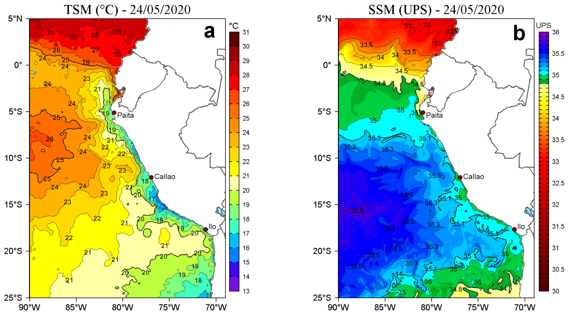
Figura 2. a) Temperatura superficial del mar (TSM, °C) y b) Salinidad superficial del mar (SSM, UPS), para el 24 de mayo de 2020. Datos: OSTIA-UKMO-L4-GLOB-v2.0 (UK Met Office, 2012; Donlon et al, 2012) disponible en https://podaac.jpl.nasa.gov/dataset/OSTIA-UKMO-L4-GLOB-v2.0 para (a) y Hybrid Coordinate Ocean Model v. GOFS 3.1 (HYCOM; Halliwell et al., 1998; 2000; Bleck, 2001) para (b). Procesamiento: LHFM/AFIOF/DGIOCC/IMARPE.
