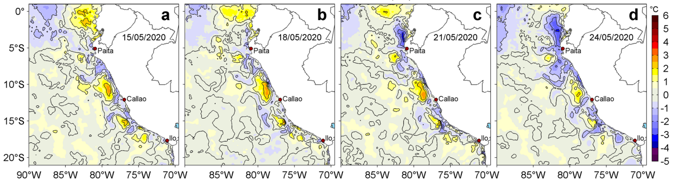
Figura 3. Anomalías de la temperatura superficial del mar (TSM, °C) para los días: a) 15, b) 18, c) 21 y d) 24 de mayo de 2020. Las anomalías se calcularon respecto de la climatología para el periodo 2007-2016. Datos: OSTIA-UKMO-L4-GLOB-v2.0 (UK Met Office, 2012; Donlon et al, 2012). Procesamiento: LHFM/AFIOF/DGIOCC/IMARPE.
