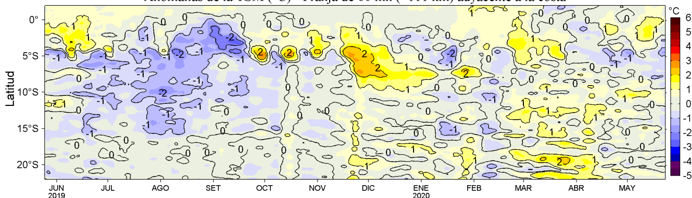
Figura 4. Variación promedio de las anomalías de la temperatura superficial del mar (TSM, °C) para una franja de 60 mn (~111 km) adyacente al litoral peruano para los últimos doce meses al 23 de mayo de 2020. Datos: OSTIA-UKMO-L4-GLOB-v2.0 (UK Met. Office, 2012; Donlon et al, 2012) disponible en https://podaac.jpl.nasa.gov/dataset/OSTIA-UKMO-L4-GLOB-v2.0 . Las anomalías se calcularon con respecto al periodo 2007-2016. Procesamiento: LHFm/AFIOF/DGIOCC/IMARPE.
