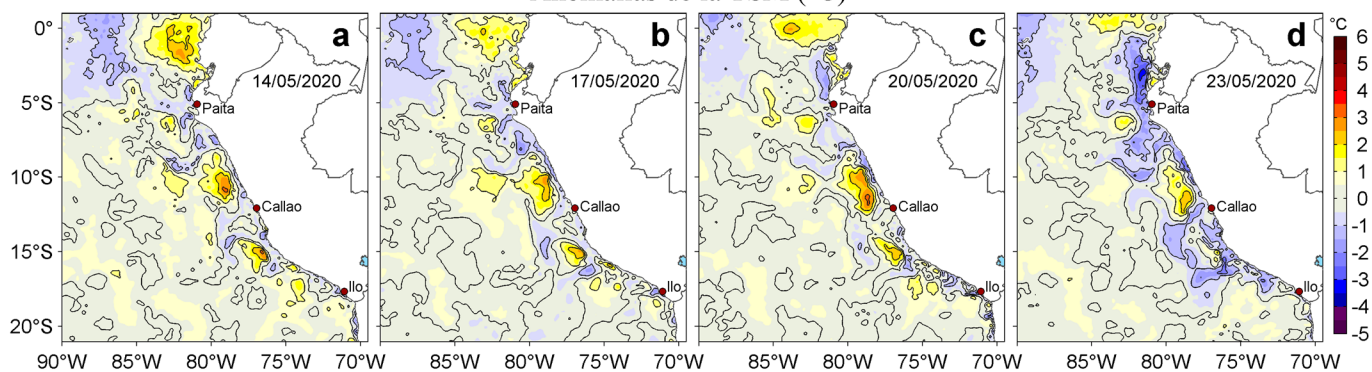
Figura 3. Anomalías de la temperatura superficial del mar (TSM, °C) para los días: a) 14, b) 17, c) 20 y d) 23 de mayo de 2020. Las anomalías se calcularon respecto de la climatología para el periodo 2007-2016. Datos: OSTIA-UKMO-L4-GLOB-v2.0 (UK Met Office, 2012; Donlon et al, 2012). Procesamiento: LHFm/AFIOF/DGIOCC/IMARPE.
