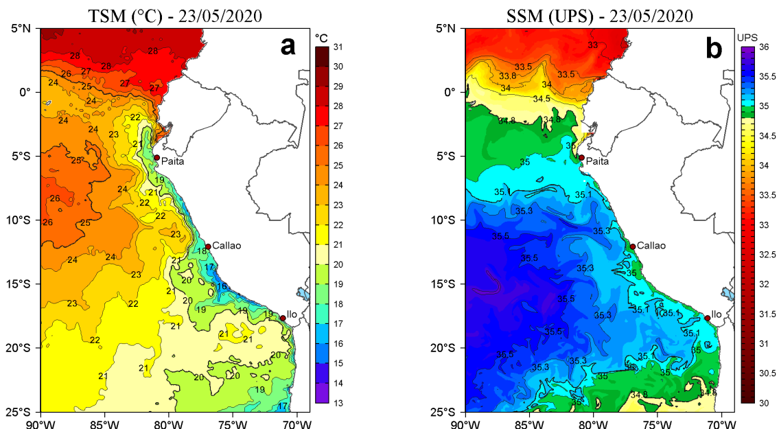
Figura 2. a) Temperatura superficial del mar (TSM, °C) y b) Salinidad superficial del mar (SSM, UPS), para el 23 de mayo de 2020. Datos: OSTIA-UKMO-L4-GLOB-v2.0 (UK Met Office, 2012; Donlon et al, 2012) disponible en https://podaac.jpl.nasa.gov/dataset/OSTIA-UKMO-L4-GLOB-v2.0 para (a) y Hybrid Coordinate Ocean Model v. GOFS 3.1 (HYCOM; Halliwell et al., 1998; 2000; Bleck, 2001) para (b). Procesamiento: LHFm/AFIOF/DGIOCC/IMARPE.
