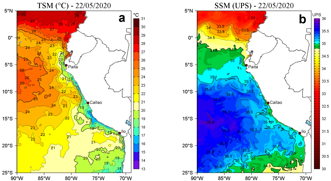
Figura 2. a) Temperatura superficial del mar (TSM, °C) y b) Salinidad superficial del mar (SSM, UPS), para el 22 de mayo de 2020. Datos: OSTIA-UKMO-L4-GLOB-v2.0 (UK Met Office, 2012; Donlon et al, 2012) disponible en https://podaac.jpl.nasa.gov/dataset/OSTIA-UKMO-L4-GLOB-v2.0 para (a) y Hybrid Coordinate Ocean Model v. GOFS 3.1 (HYCOM; Halliwell et al., 1998; 2000; Bleck, 2001) para (b). Procesamiento: LHFM/AFIOF/DGIOCC/IMARPE.
