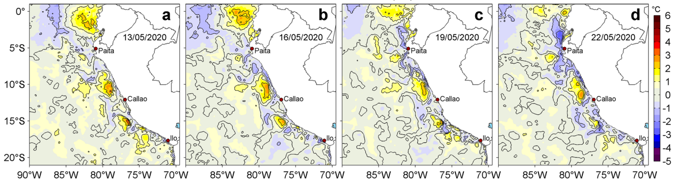
Figura 3. Anomalías de la temperatura superficial del mar (TSM, °C) para los días: a) 13, b) 16, c) 19 y d) 22 de mayo de 2020. Las anomalías se calcularon respecto de la climatología para el periodo 2007-2016. Datos: OSTIA-UKMO-L4-GLOB-v2.0 (UK Met Office, 2012; Donlon et al, 2012). Procesamiento: LHFM/AFIOF/DGIOCC/IMARPE.
