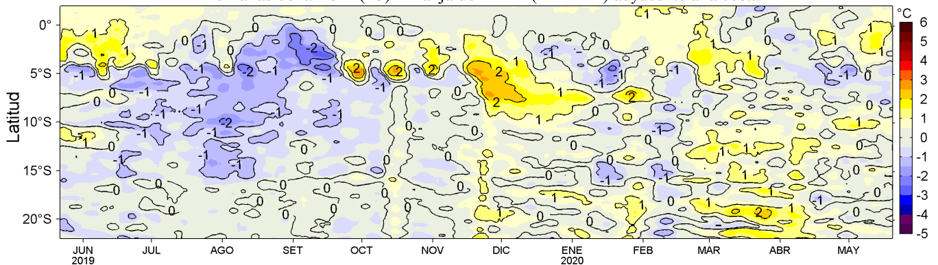
Figura 4. Variación promedio de las anomalías de la temperatura superficial del mar (TSM, °C) para una franja de 60 mn (~111 km) adyacente al litoral peruano para los últimos doce meses al 20 de mayo de 2020. Datos: OSTIA-UKMO-L4-GLOB-v2.0 (UK Met. Office, 2012; Donlon et al, 2012) disponible en https://podaac.jpl.nasa.gov/dataset/OSTIA-UKMO-L4-GLOB-v2.0 . Las anomalías se calcularon con respecto al periodo 2007-2016. Procesamiento: LHF/AFIOF/DGIOCC/IMARPE.
