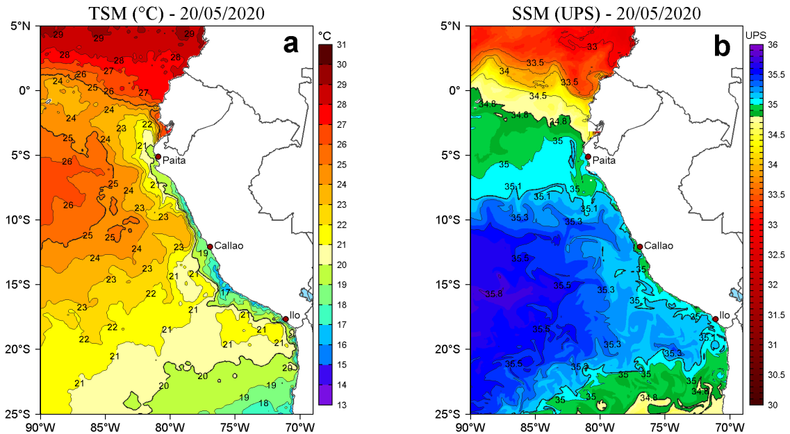
Figura 2. a) Temperatura superficial del mar (TSM, °C) y b) Salinidad superficial del mar (SSM, UPS), para el 20 de mayo de 2020. Datos: OSTIA-UKMO-L4-GLOB-v2.0 (UK Met Office, 2012; Donlon et al, 2012) disponible en https://podaac.jpl.nasa.gov/dataset/OSTIA-UKMO-L4-GLOB-v2.0 para (a) y Hybrid Coordinate Ocean Model v. GOFS 3.1 (HYCOM; Halliwell et al., 1998; 2000; Bleck, 2001) para (b). Procesamiento: LHF/AFIOF/DGIOCC/IMARPE.
