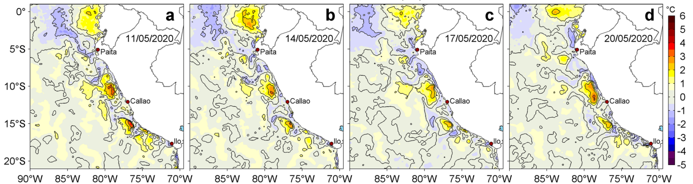
Figura 3. Anomalías de la temperatura superficial del mar (TSM, °C) para los días: a) 11, b) 14, c) 17 y d) 20 de mayo de 2020. Las anomalías se calcularon respecto de la climatología para el periodo 2007-2016. Datos: OSTIA-UKMO-L4-GLOB-v2.0 (UK Met Office, 2012; Donlon et al, 2012). Procesamiento: LHF/AFIOF/DGIOCC/IMARPE.
