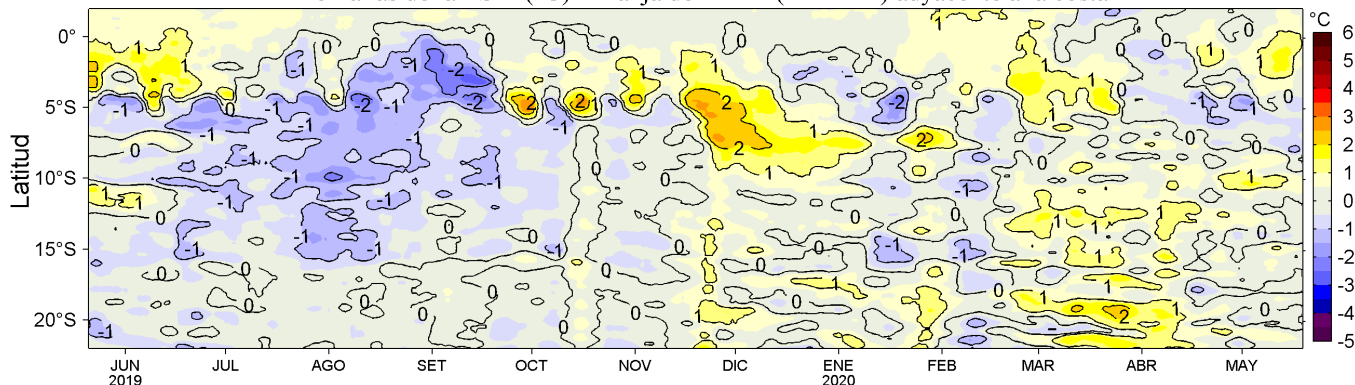
Figura 4. Variación promedio de las anomalías de la temperatura superficial del mar (TSM, °C) para una franja de 60 mn (~111 km) adyacente al litoral peruano para los últimos doce meses al 19 de mayo de 2020. Datos: OSTIA-UKMO-L4-GLOB-v2.0 (UK Met. Office, 2012; Donlon et al, 2012) disponible en https://podaac.jpl.nasa.gov/dataset/OSTIA-UKMO-L4-GLOB-v2.0 . Las anomalías se calcularon con respecto al periodo 2007-2016. Procesamiento: LHF/AFIOF/DGIOCC/IMARPE.
