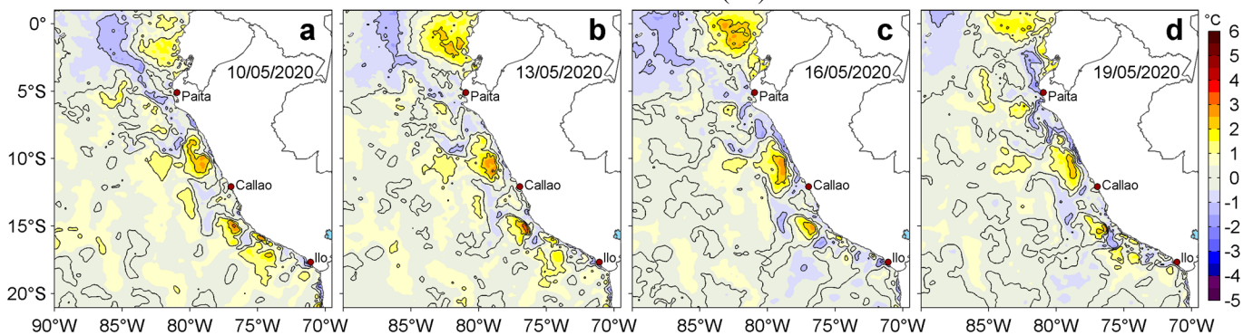
Figura 3. Anomalías de la temperatura superficial del mar (TSM, °C) para los días: a) 10, b) 13, c) 16 y d) 19 de mayo de 2020. Las anomalías se calcularon respecto de la climatología para el periodo 2007-2016. Datos: OSTIA-UKMO-L4-GLOB-v2.0 (UK Met Office, 2012; Donlon et al, 2012). Procesamiento: LHF/AFIOF/DGIOCC/IMARPE.
