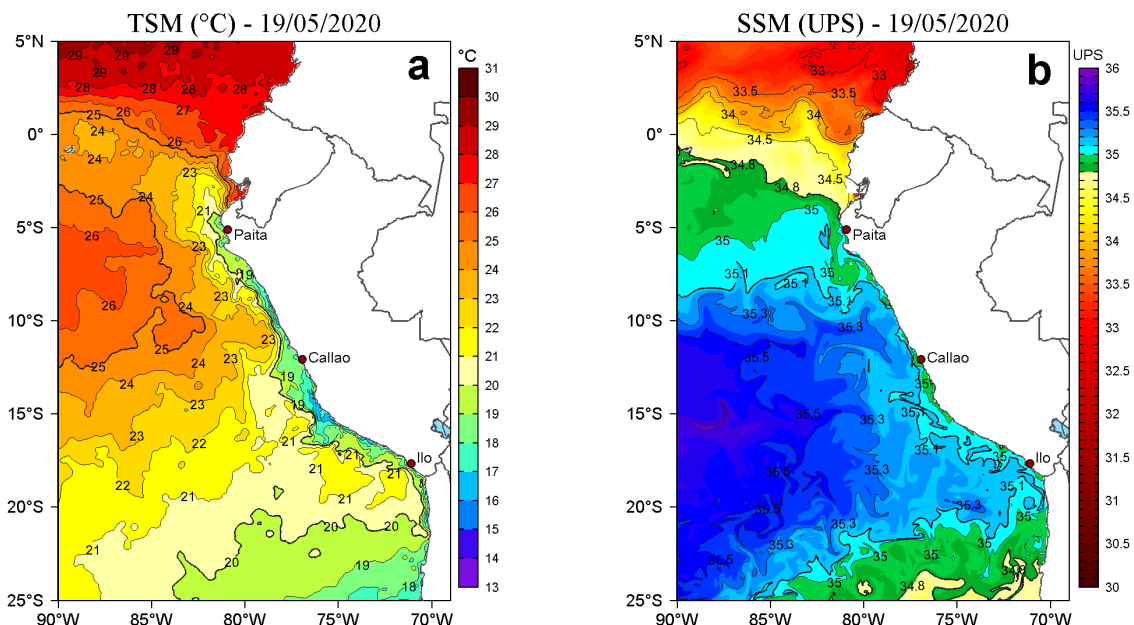
Figura 2. a) Temperatura superficial del mar (TSM, °C) y b) Salinidad superficial del mar (SSM, UPS), para el 19 de mayo de 2020. Datos: OSTIA-UKMO-L4-GLOB-v2.0 (UK Met Office, 2012; Donlon et al, 2012) disponible en https://podaac.jpl.nasa.gov/dataset/OSTIA-UKMO-L4-GLOB-v2.0 para (a) y Hybrid Coordinate Ocean Model v. GOFS 3.1 (HYCOM; Halliwell et al., 1998; 2000; Bleck, 2001) para (b). Procesamiento: LHF/AFIOF/DGIOCC/IMARPE.
