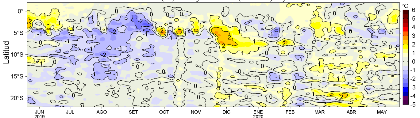
Figura 4. Variación promedio de las anomalías de la temperatura superficial del mar (TSM, °C) para una franja de 60 mn (~111 km) adyacente al litoral peruano para los últimos doce meses al 18 de mayo de 2020. Datos: OSTIA-UKMO-L4-GLOB-v2.0 (UK Met. Office, 2012; Donlon et al, 2012) disponible en https://podaac.jpl.nasa.gov/dataset/OSTIA-UKMO-L4-GLOB-v2.0 . Las anomalías se calcularon con respecto al periodo 2007-2016. Procesamiento: LHF/AFIOF/DGIOCC/IMARPE.
