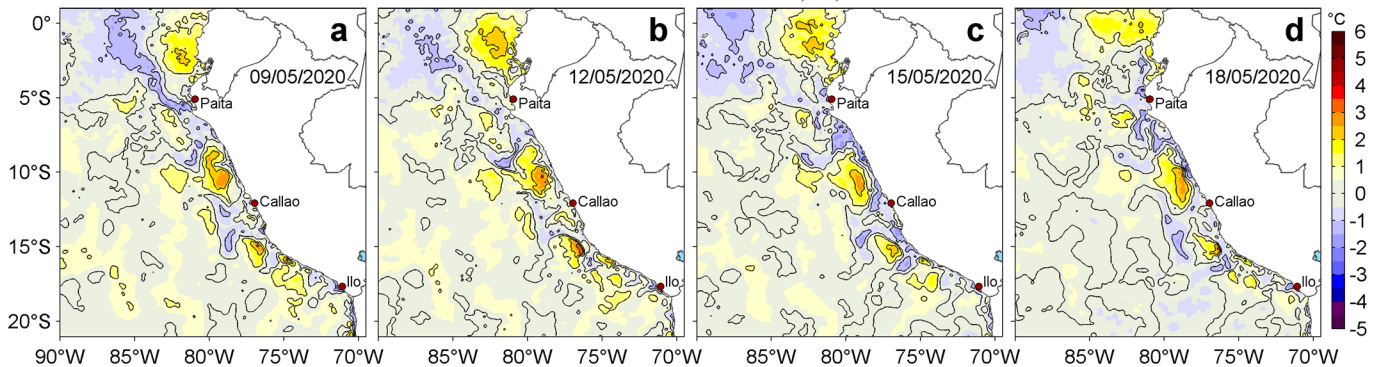
Figura 3. Anomalías de la temperatura superficial del mar (TSM, °C) para los días: a) 09, b) 12, c) 15 y d) 18 de mayo de 2020. Las anomalías se calcularon respecto de la climatología para el periodo 2007-2016. Datos: OSTIA-UKMO-L4-GLOB-v2.0 (UK Met Office, 2012; Donlon et al, 2012). Procesamiento: LHF/AFIOF/DGIOCC/IMARPE.
