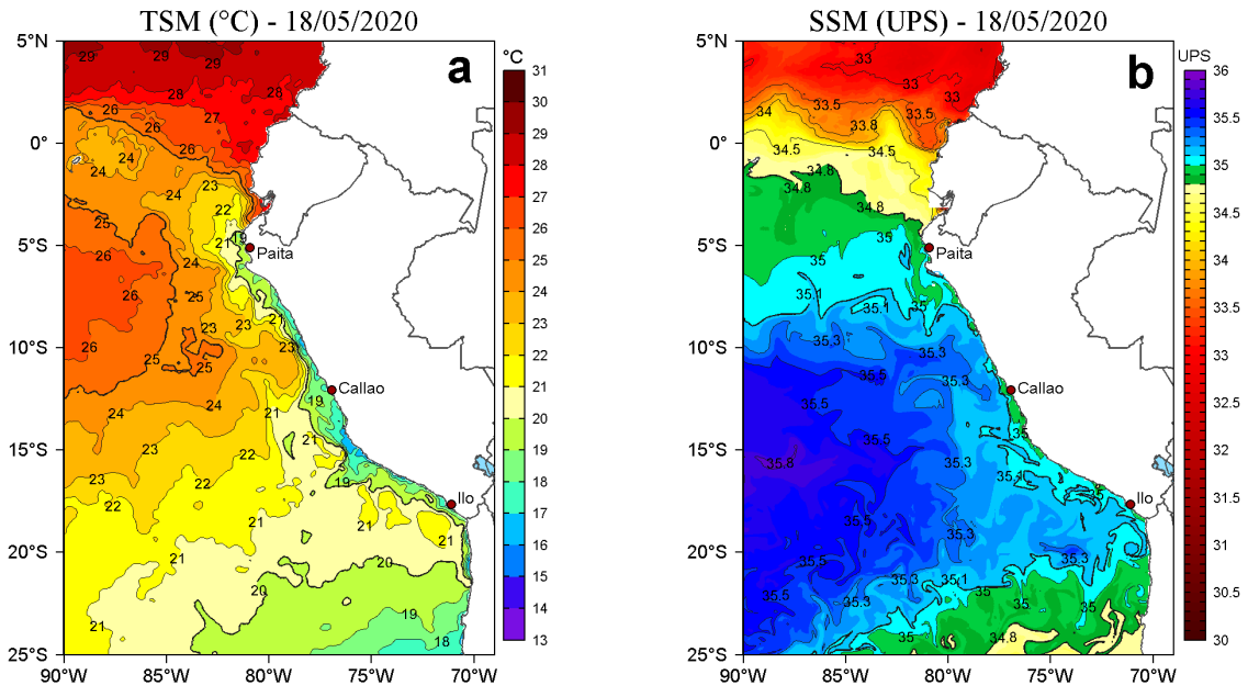
Figura 2. a) Temperatura superficial del mar (TSM, °C) y b) Salinidad superficial del mar (SSM, UPS), para el 18 de mayo de 2020. Datos: OSTIA-UKMO-L4-GLOB-v2.0 (UK Met Office, 2012; Donlon et al, 2012) disponible en https://podaac.jpl.nasa.gov/dataset/OSTIA-UKMO-L4-GLOB-v2.0 para (a) y Hybrid Coordinate Ocean Model v. GOFS 3.1 (HYCOM; Halliwell et al., 1998; 2000; Bleck, 2001) para (b). Procesamiento: LHF/AFIOF/DGIOCC/IMARPE.
