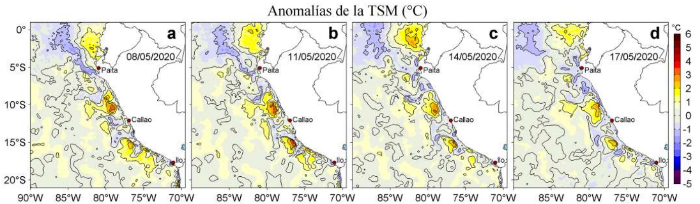
Figura 3. Anomalías de la temperatura superficial del mar (TSM, °C) para los días: a) 08, b) 11, c) 14 y d) 17 de mayo de 2020. Las anomalías se calcularon respecto de la climatología para el periodo 2007-2016. Datos: OSTIA-UKMO-L4-GLOB-v2.0 (UK Met Office, 2012; Donlon et al, 2012). Procesamiento: LHFH/AFIOF/DGIOCC/IMARPE.
