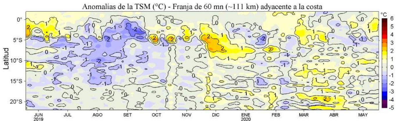
Figura 4. Variación promedio de las anomalías de la temperatura superficial del mar (TSM, °C) para una franja de 60 mn (~111 km) adyacente al litoral peruano para los últimos doce meses al 17 de mayo de 2020. Datos: OSTIA-UKMO-L4-GLOB-v2.0 (UK Met. Office, 2012; Donlon et al, 2012) disponible en https://podaac.jpl.nasa.gov/dataset/OSTIA-UKMO-L4-GLOB-v2.0 . Las anomalías se calcularon con respecto al periodo 2007-2016. Procesamiento: LHFH/AFIOF/DGIOCC/IMARPE.
