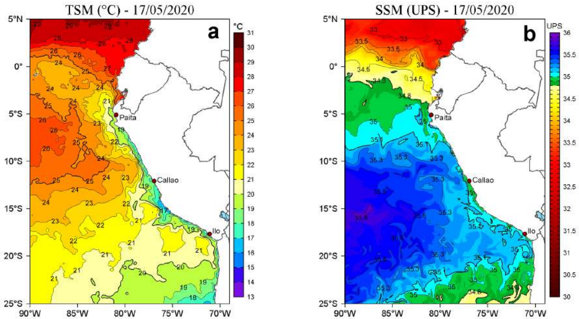
Figura 2. a) Temperatura superficial del mar (TSM, °C) y b) Salinidad superficial del mar (SSM, UPS), para el 17 de mayo de 2020. Datos: OSTIA-UKMO-L4-GLOB-v2.0 (UK Met Office, 2012; Donlon et al, 2012) disponible en https://podaac.jpl.nasa.gov/dataset/OSTIA-UKMO-L4-GLOB-v2.0 para (a) y Hybrid Coordinate Ocean Model v. GOFS 3.1 (HYCOM; Halliwell et al., 1998; 2000; Bleck, 2001) para (b). Procesamiento: LHFH/AFIOF/DGIOCC/IMARPE.
