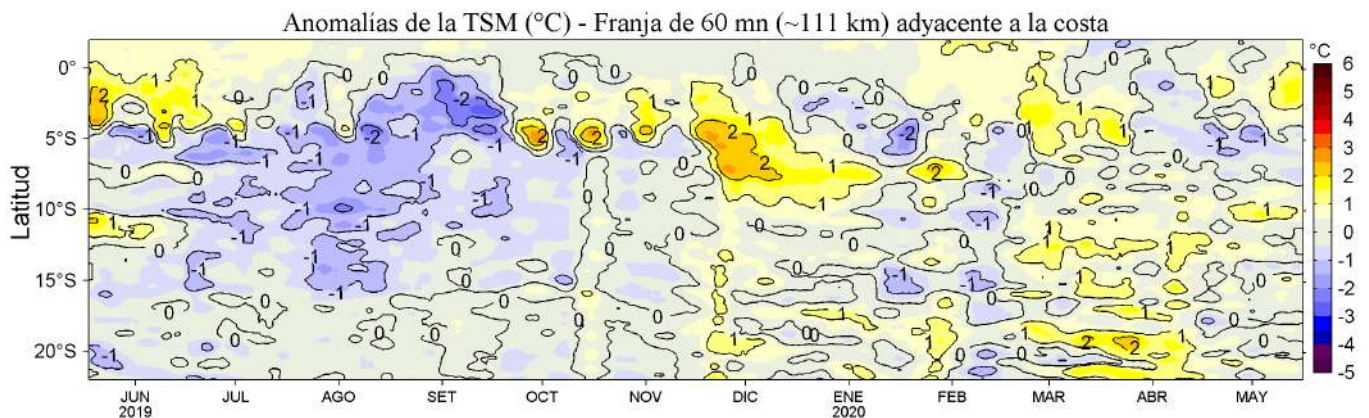
Figura 4. Variación promedio de las anomalías de la temperatura superficial del mar (TSM, °C) para una franja de 60 mn (~111 km) adyacente al litoral peruano para los últimos doce meses al 16 de mayo de 2020. Datos: OSTIA-UKMO-L4-GLOB-v2.0 (UK Met. Office, 2012; Donlon et al, 2012) disponible en https://podaac.jpl.nasa.gov/dataset/OSTIA-UKMO-L4-GLOB-v2.0 . Las anomalías se calcularon con respecto al periodo 2007-2016. Procesamiento: LHF/AFIOF/DGIOCC/IMARPE.
