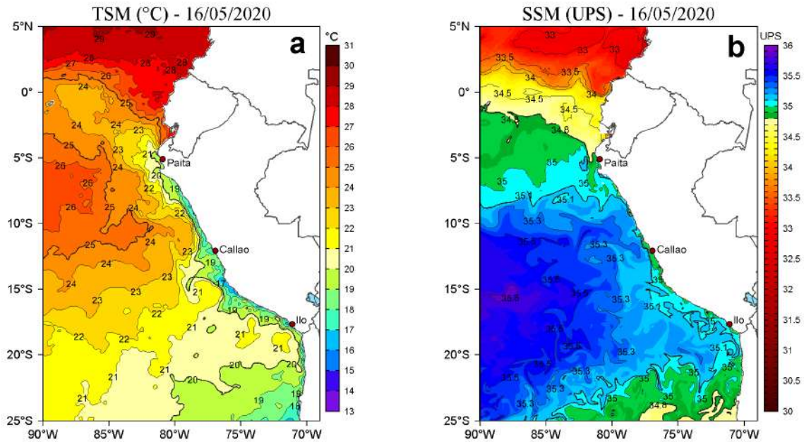
Figura 2. a) Temperatura superficial del mar (TSM, °C) y b) Salinidad superficial del mar (SSM, UPS), para el 16 de mayo de 2020. Datos: OSTIA-UKMO-L4-GLOB-v2.0 (UK Met Office, 2012; Donlon et al, 2012) disponible en https://podaac.jpl.nasa.gov/dataset/OSTIA-UKMO-L4-GLOB-v2.0 para (a) y Hybrid Coordinate Ocean Model v. GOFS 3.1 (HYCOM; Halliwell et al., 1998; 2000; Bleck, 2001) para (b). Procesamiento: LHF/AFIOF/DGIOCC/IMARPE.
