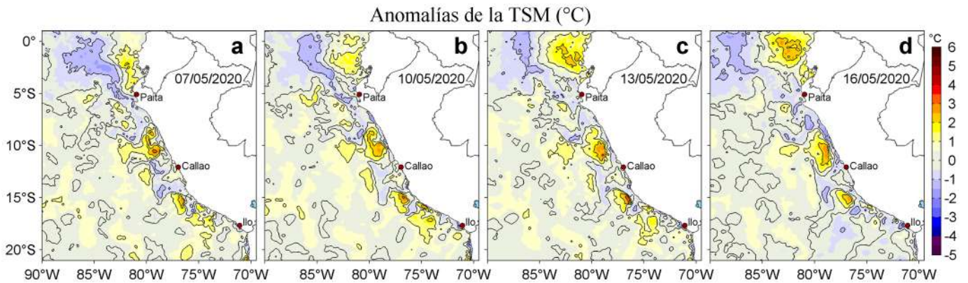
Figura 3. Anomalías de la temperatura superficial del mar (TSM, °C) para los días: a) 07, b) 10, c) 13 y d) 16 de mayo de 2020. Las anomalías se calcularon respecto de la climatología para el periodo 2007-2016. Datos: OSTIA-UKMO-L4-GLOB-v2.0 (UK Met Office, 2012; Donlon et al, 2012). Procesamiento: LHF/AFIOF/DGIOCC/IMARPE.
