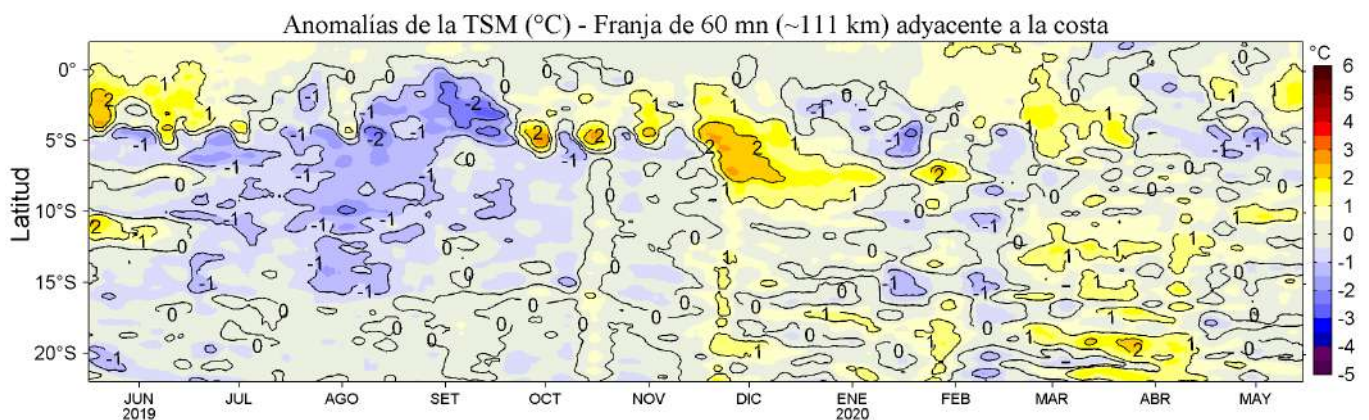
Figura 4. Variación promedio de las anomalías de la temperatura superficial del mar (TSM, °C) para una franja de 60 mn (~111 km) adyacente al litoral peruano para los últimos doce meses al 15 de mayo de 2020. Datos: OSTIA-UKMO-L4-GLOB-v2.0 (UK Met. Office, 2012; Donlon et al, 2012) disponible en https://podaac.jpl.nasa.gov/dataset/OSTIA-UKMO-L4-GLOB-v2.0 . Las anomalías se calcularon con respecto al periodo 2007-2016. Procesamiento: LHF/AFIOF/DGIOCC/IMARPE.
