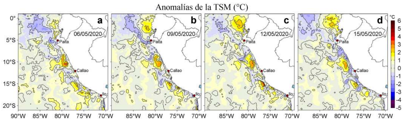
Figura 3. Anomalías de la temperatura superficial del mar (TSM, °C) para los días: a) 06, b) 09, c) 12 y d) 15 de mayo de 2020. Las anomalías se calcularon respecto de la climatología para el periodo 2007-2016. Datos: OSTIA-UKMO-L4-GLOB-v2.0 (UK Met Office, 2012; Donlon et al, 2012). Procesamiento: LHF/AFIOF/DGIOCC/IMARPE.
