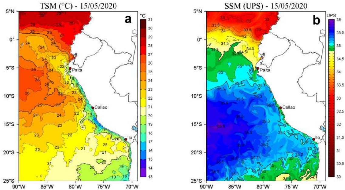
Figura 2. a) Temperatura superficial del mar (TSM, °C) y b) Salinidad superficial del mar (SSM, UPS), para el 15 de mayo de 2020. Datos: OSTIA-UKMO-L4-GLOB-v2.0 (UK Met Office, 2012; Donlon et al, 2012) disponible en https://podaac.jpl.nasa.gov/dataset/OSTIA-UKMO-L4-GLOB-v2.0 para (a) y Hybrid Coordinate Ocean Model v. GOFS 3.1 (HYCOM; Halliwell et al., 1998; 2000; Bleck, 2001) para (b). Procesamiento: LHF/AFIOF/DGIOCC/IMARPE.
