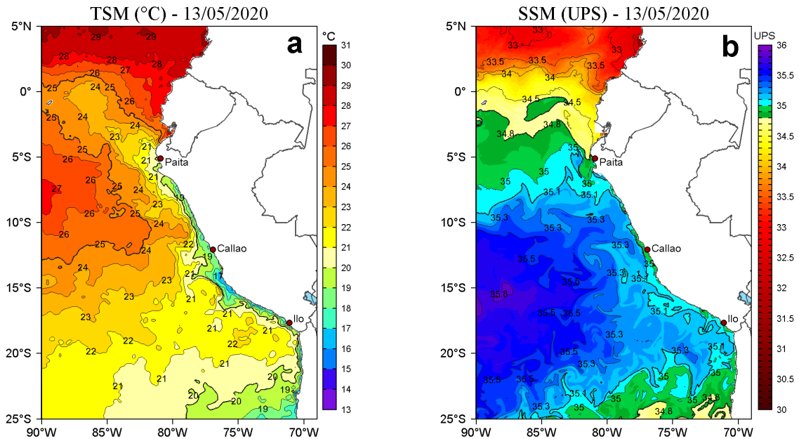
Figura 2. a) Temperatura superficial del mar (TSM, °C) y b) Salinidad superficial del mar (SSM, UPS), para el 13 de mayo de 2020. Datos: OSTIA-UKMO-L4-GLOB-v2.0 (UK Met Office, 2012; Donlon et al, 2012) disponible en https://podaac.jpl.nasa.gov/dataset/OSTIA-UKMO-L4-GLOB-v2.0 para (a) y Hybrid Coordinate Ocean Model v. GOFS 3.1 (HYCOM; Halliwell et al., 1998; 2000; Bleck, 2001) para (b). Procesamiento: LHFM/AFIOF/DGIOCC/IMARPE.
