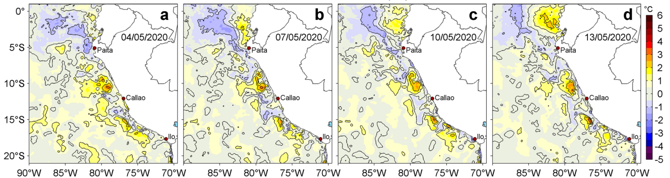
Figura 3. Anomalías de la temperatura superficial del mar (TSM, °C) para los días: a) 04, b) 07, c) 10 y d) 13 de mayo de 2020. Las anomalías se calcularon respecto de la climatología para el periodo 2007-2016. Datos: OSTIA-UKMO-L4-GLOB-v2.0 (UK Met Office, 2012; Donlon et al, 2012). Procesamiento: LHFM/AFIOF/DGIOCC/IMARPE.
