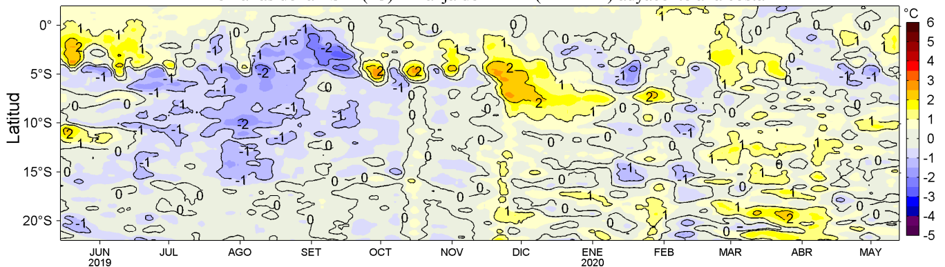
Figura 4. Variación promedio de las anomalías de la temperatura superficial del mar (TSM, °C) para una franja de 60 mn (~111 km) adyacente al litoral peruano para los últimos doce meses al 13 de mayo de 2020. Datos: OSTIA-UKMO-L4-GLOB-v2.0 (UK Met. Office, 2012; Donlon et al, 2012) disponible en https://podaac.jpl.nasa.gov/dataset/OSTIA-UKMO-L4-GLOB-v2.0 . Las anomalías se calcularon con respecto al periodo 2007-2016. Procesamiento: LHFM/AFIOF/DGIOCC/IMARPE.
