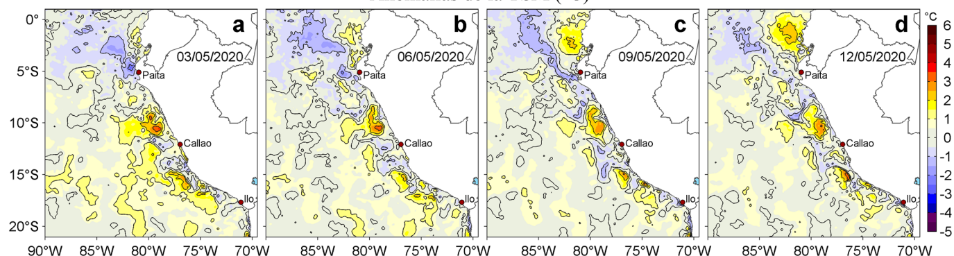
Figura 3. Anomalías de la temperatura superficial del mar (TSM, °C) para los días: a) 03, b) 06, c) 09 y d) 12 de mayo de 2020. Las anomalías se calcularon respecto de la climatología para el periodo 2007-2016. Datos: OSTIA-UKMO-L4-GLOB-v2.0 (UK Met Office, 2012; Donlon et al, 2012). Procesamiento: LHF/M/AFIOF/DGIOCC/IMARPE.
