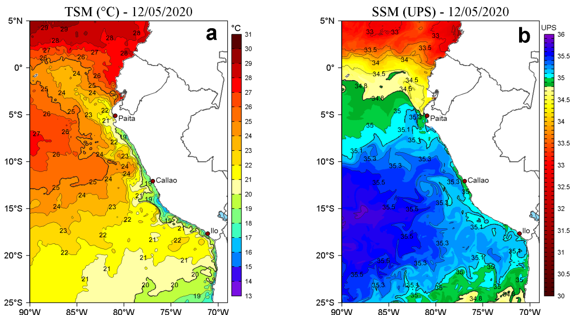
Figura 2. a) Temperatura superficial del mar (TSM, °C) y b) Salinidad superficial del mar (SSM, UPS), para el 12 de mayo de 2020. Datos: OSTIA-UKMO-L4-GLOB-v2.0 (UK Met Office, 2012; Donlon et al, 2012) disponible en https://podaac.jpl.nasa.gov/dataset/OSTIA-UKMO-L4-GLOB-v2.0 para (a) y Hybrid Coordinate Ocean Model v. GOFS 3.1 (HYCOM; Halliwell et al., 1998; 2000; Bleck, 2001) para (b). Procesamiento: LHF/M/AFIOF/DGIOCC/IMARPE.
