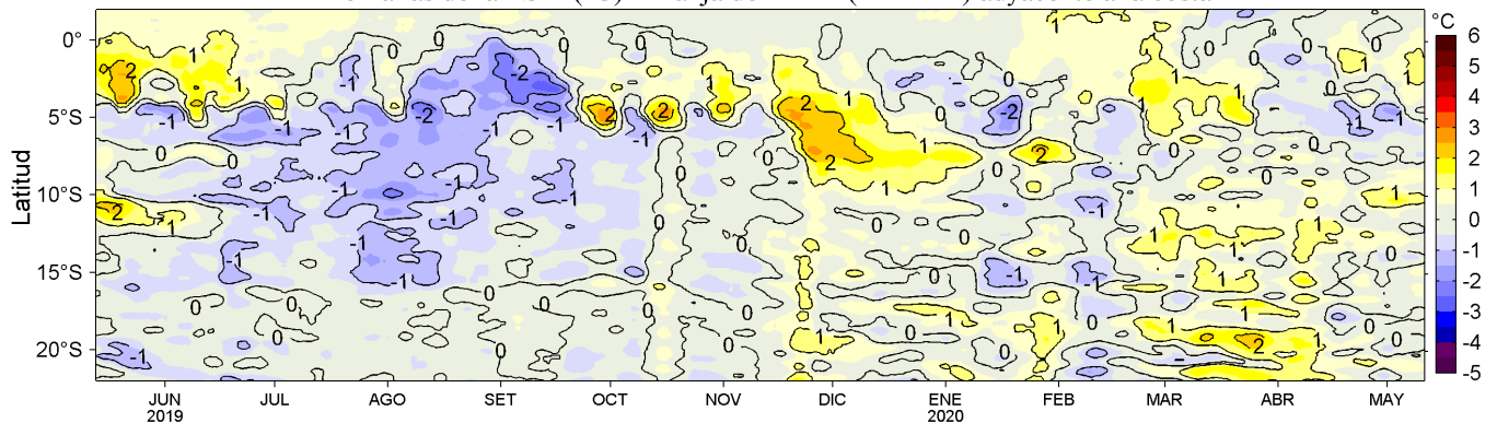
Figura 4. Variación promedio de las anomalías de la temperatura superficial del mar (TSM, °C) para una franja de 60 mn (~111 km) adyacente al litoral peruano para los últimos doce meses al 11 de mayo de 2020. Datos: OSTIA-UKMO-L4-GLOB-v2.0 (UK Met. Office, 2012; Donlon et al, 2012) disponible en https://podaac.jpl.nasa.gov/dataset/OSTIA-UKMO-L4-GLOB-v2.0 . Las anomalías se calcularon con respecto al periodo 2007-2016. Procesamiento: LHF/AFIOF/DGIOCC/IMARPE.
