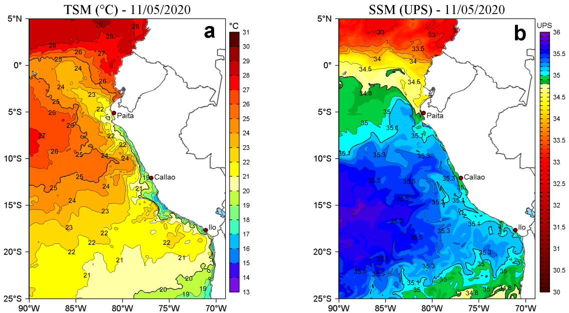
Figura 2. a) Temperatura superficial del mar (TSM, °C) y b) Salinidad superficial del mar (SSM, UPS), para el 11 de mayo de 2020. Datos: OSTIA-UKMO-L4-GLOB-v2.0 (UK Met Office, 2012; Donlon et al, 2012) disponible en https://podaac.jpl.nasa.gov/dataset/OSTIA-UKMO-L4-GLOB-v2.0 para (a) y Hybrid Coordinate Ocean Model v. GOFS 3.1 (HYCOM; Halliwell et al., 1998; 2000; Bleck, 2001) para (b). Procesamiento: LHF/AFIOF/DGIOCC/IMARPE.
