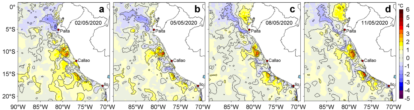
Figura 3. Anomalías de la temperatura superficial del mar (TSM, °C) para los días: a) 02, b) 05, c) 08 y d) 11 de mayo de 2020. Las anomalías se calcularon respecto de la climatología para el periodo 2007-2016. Datos: OSTIA-UKMO-L4-GLOB-v2.0 (UK Met Office, 2012; Donlon et al, 2012). Procesamiento: LHF/AFIOF/DGIOCC/IMARPE.
