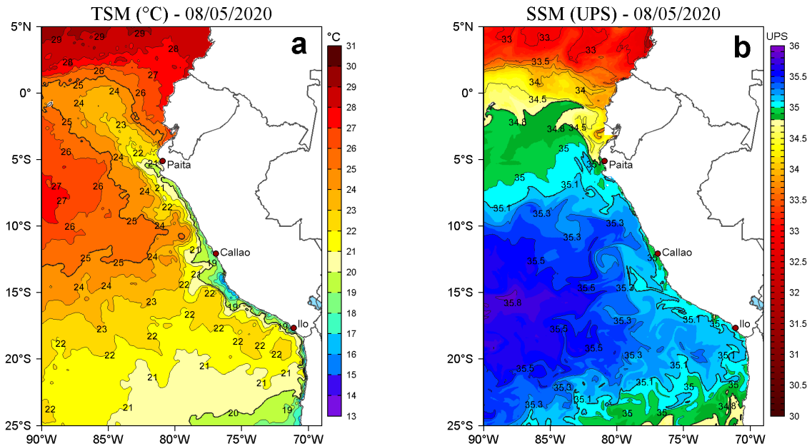
Figura 2. a) Temperatura superficial del mar (TSM, °C) y b) Salinidad superficial del mar (SSM, UPS), para el 08 de mayo de 2020. Datos: OSTIA-UKMO-L4-GLOB-v2.0 (UK Met Office, 2012; Donlon et al, 2012) disponible en https://podaac.jpl.nasa.gov/dataset/OSTIA-UKMO-L4-GLOB-v2.0 para (a) y Hybrid Coordinate Ocean Model v. GOFS 3.1 (HYCOM; Halliwell et al., 1998; 2000; Bleck, 2001) para (b). Procesamiento: LHF/AFIOF/DGIOCC/IMARPE.
