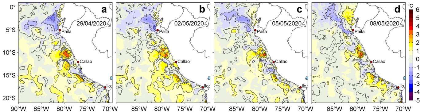
Figura 3. Anomalías de la temperatura superficial del mar (TSM, °C) para los días: a) 29 de abril, b) 02, c) 05 y d) 08 de mayo de 2020. Las anomalías se calcularon respecto de la climatología para el periodo 2007-2016. Datos: OSTIA-UKMO-L4-GLOB-v2.0 (UK Met Office, 2012; Donlon et al, 2012). Procesamiento: LHF/AFIOF/DGIOCC/IMARPE.
