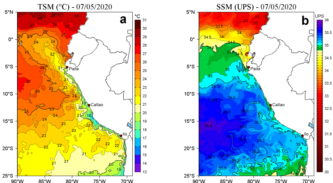
Figura 2. a) Temperatura superficial del mar (TSM, °C) y b) Salinidad superficial del mar (SSM, UPS), para el 07 de mayo de 2020. Datos: OSTIA-UKMO-L4-GLOB-v2.0 (UK Met Office, 2012; Donlon et al, 2012) disponible en https://podaac.jpl.nasa.gov/dataset/OSTIA-UKMO-L4-GLOB-v2.0 para (a) y Hybrid Coordinate Ocean Model v. GOFS 3.1 (HYCOM; Halliwell et al., 1998; 2000; Bleck, 2001) para (b). Procesamiento: LHFM/AFIOF/DGIOCC/IMARPE.
