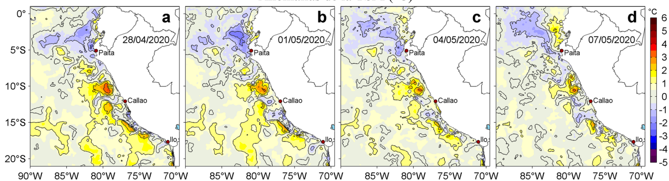
Figura 3. Anomalías de la temperatura superficial del mar (TSM, °C) para los días: a) 28 de abril, b) 01, c) 04 y d) 07 de mayo de 2020. Las anomalías se calcularon respecto de la climatología para el periodo 2007-2016. Datos: OSTIA-UKMO-L4-GLOB-v2.0 (UK Met Office, 2012; Donlon et al, 2012). Procesamiento: LHFM/AFIOF/DGIOCC/IMARPE.
