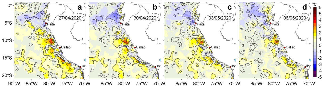
Figura 3. Anomalías de la temperatura superficial del mar (TSM, °C) para los días: a) 27 y b) 30 de abril, c) 03 y d) 06 de mayo de 2020. Las anomalías se calcularon respecto de la climatología para el periodo 2007-2016. Datos: OSTIA-UKMO-L4-GLOB-v2.0 (UK Met Office, 2012; Donlon et al, 2012). Procesamiento: LHF/AFIOF/DGIOCC/IMARPE.
