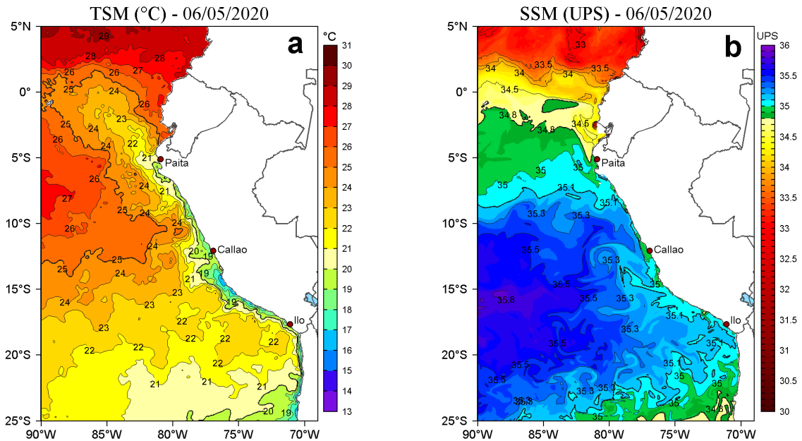
Figura 2. a) Temperatura superficial del mar (TSM, °C) y b) Salinidad superficial del mar (SSM, UPS), para el 06 de mayo de 2020. Datos: OSTIA-UKMO-L4-GLOB-v2.0 (UK Met Office, 2012; Donlon et al, 2012) disponible en https://podaac.jpl.nasa.gov/dataset/OSTIA-UKMO-L4-GLOB-v2.0 para (a) y Hybrid Coordinate Ocean Model v. GOFS 3.1 (HYCOM; Halliwell et al., 1998; 2000; Bleck, 2001) para (b). Procesamiento: LHF/AFIOF/DGIOCC/IMARPE.
