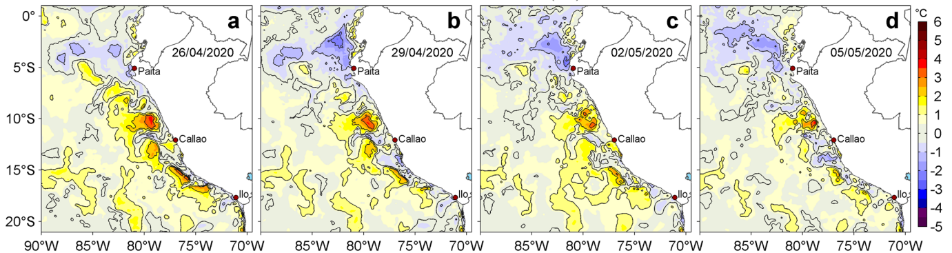
Figura 3. Anomalías de la temperatura superficial del mar (TSM, °C) para los días: a) 26 y b) 29 de abril, c) 02 y d) 05 de mayo de 2020. Las anomalías se calcularon respecto de la climatología para el periodo 2007-2016. Datos: OSTIA-UKMO-L4-GLOB-v2.0 (UK Met Office, 2012; Donlon et al, 2012). Procesamiento: LHF/AFIOF/DGIOCC/IMARPE.
