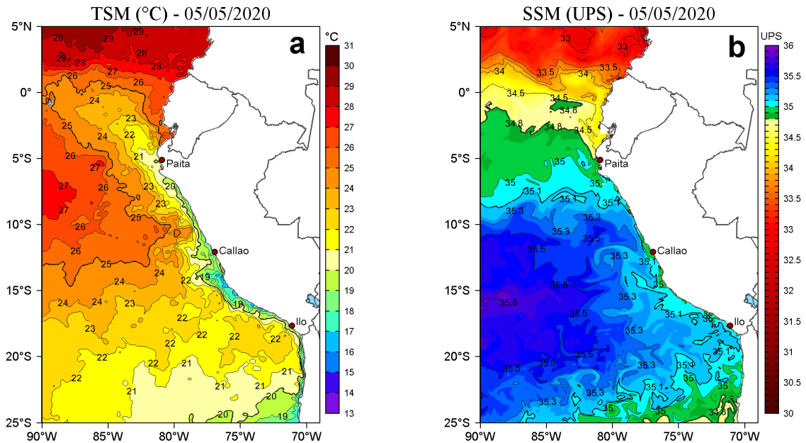
Figura 2. a) Temperatura superficial del mar (TSM, °C) y b) Salinidad superficial del mar (SSM, UPS), para el 05 de mayo de 2020. Datos: OSTIA-UKMO-L4-GLOB-v2.0 (UK Met Office, 2012; Donlon et al, 2012) disponible en https://podaac.jpl.nasa.gov/dataset/OSTIA-UKMO-L4-GLOB-v2.0 para (a) y Hybrid Coordinate Ocean Model v. GOFS 3.1 (HYCOM; Halliwell et al., 1998; 2000; Bleck, 2001) para (b). Procesamiento: LHF/AFIOF/DGIOCC/IMARPE.
