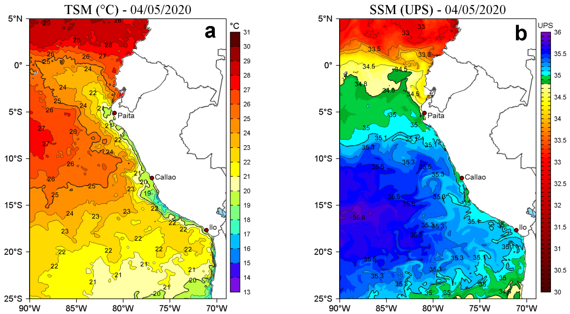
Figura 2. a) Temperatura superficial del mar (TSM, °C) y b) Salinidad superficial del mar (SSM, UPS), para el 04 de mayo de 2020. Datos: OSTIA-UKMO-L4-GLOB-v2.0 (UK Met Office, 2012; Donlon et al, 2012) disponible en https://podaac.jpl.nasa.gov/dataset/OSTIA-UKMO-L4-GLOB-v2.0 para (a) y Hybrid Coordinate Ocean Model v. GOFS 3.1 (HYCOM; Halliwell et al., 1998; 2000; Bleck, 2001) para (b). Procesamiento: LHF/AFIOF/DGIOCC/IMARPE.
