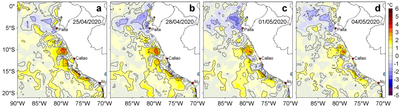
Figura 3. Anomalías de la temperatura superficial del mar (TSM, °C) para los días: a) 25 y b) 28 de abril, c) 01 y d) 04 de mayo de 2020. Las anomalías se calcularon respecto de la climatología para el periodo 2007-2016. Datos: OSTIA-UKMO-L4-GLOB-v2.0 (UK Met Office, 2012; Donlon et al, 2012). Procesamiento: LHF/AFIOF/DGIOCC/IMARPE.
