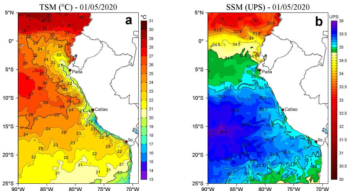
Figura 2. a) Temperatura superficial del mar (TSM, °C) y b) Salinidad superficial del mar (SSM, UPS), para el 01 de mayo de 2020. Datos: OSTIA-UKMO-L4-GLOB-v2.0 (UK Met Office, 2012; Donlon et al, 2012) disponible en https://podaac.jpl.nasa.gov/dataset/OSTIA-UKMO-L4-GLOB-v2.0 para (a) y Hybrid Coordinate Ocean Model v. GOFS 3.1 (HYCOM; Halliwell et al., 1998; 2000; Bleck, 2001) para (b). Procesamiento: LHFm/AFIOF/DGIOCC/IMARPE.
