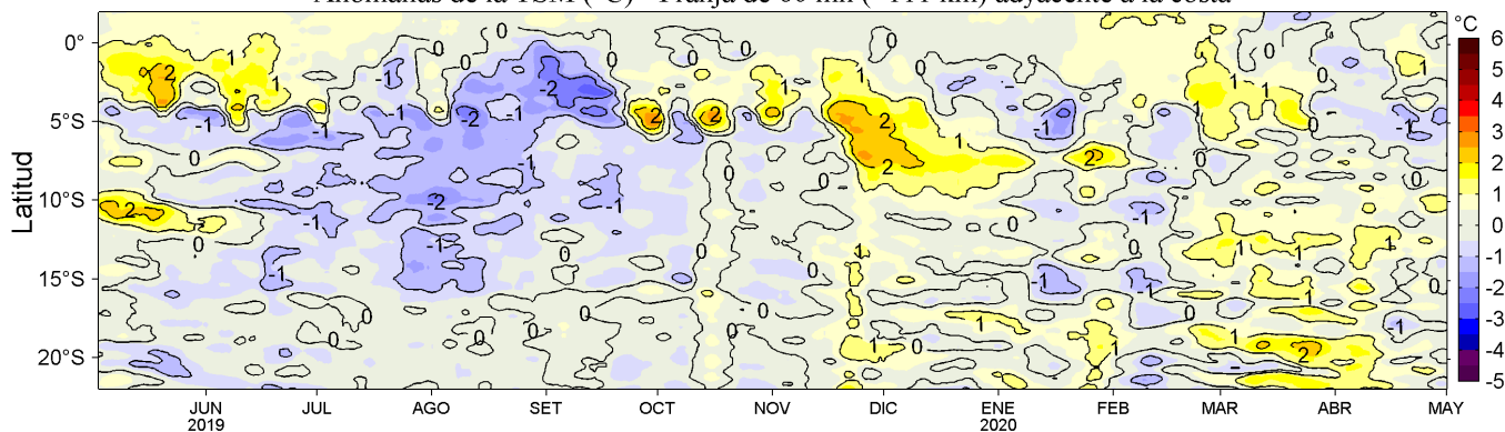
Figura 4. Variación promedio de las anomalías de la temperatura superficial del mar (TSM, °C) para una franja de 60 mn (~111 km) adyacente al litoral peruano para los últimos doce meses al 01 de mayo de 2020. Datos: OSTIA-UKMO-L4-GLOB-v2.0 (UK Met. Office, 2012; Donlon et al, 2012) disponible en https://podaac.jpl.nasa.gov/dataset/OSTIA-UKMO-L4-GLOB-v2.0 . Las anomalías se calcularon con respecto al periodo 2007-2016. Procesamiento: LHFm/AFIOF/DGIOCC/IMARPE.
