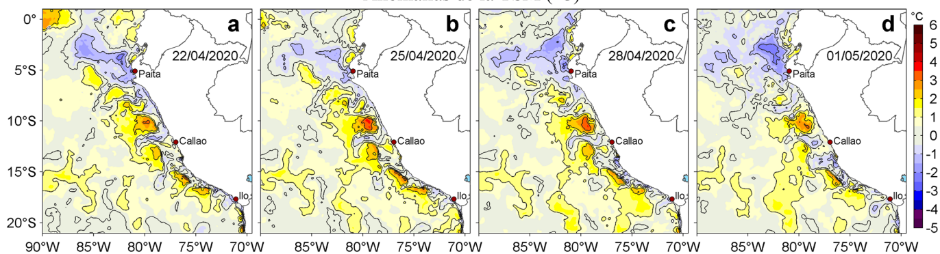
Figura 3. Anomalías de la temperatura superficial del mar (TSM, °C) para los días: a) 22, b) 25 y c) 28 de abril y d) 01 de mayo de 2020. Las anomalías se calcularon respecto de la climatología para el periodo 2007-2016. Datos: OSTIA-UKMO-L4-GLOB-v2.0 (UK Met Office, 2012; Donlon et al, 2012). Procesamiento: LHFm/AFIOF/DGIOCC/IMARPE.
