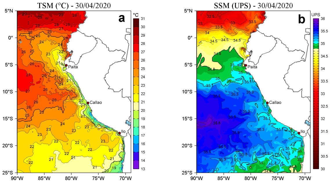
Figura 2. a) Temperatura superficial del mar (TSM, °C) y b) Salinidad superficial del mar (SSM, UPS), para el 30 de abril de 2020. Datos: OSTIA-UKMO-L4-GLOB-v2.0 (UK Met Office, 2012; Donlon et al, 2012) disponible en https://podaac.jpl.nasa.gov/dataset/OSTIA-UKMO-L4-GLOB-v2.0 para (a) y Hybrid Coordinate Ocean Model v. GOFS 3.1 (HYCOM; Halliwell et al., 1998; 2000; Bleck, 2001) para (b). Procesamiento: LHF/AFIOF/DGIOCC/IMARPE.
