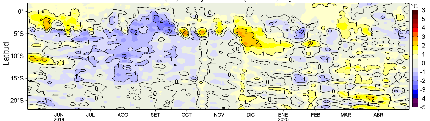
Figura 4. Variación promedio de las anomalías de la temperatura superficial del mar (TSM, °C) para una franja de 60 mn (~111 km) adyacente al litoral peruano para los últimos doce meses al 30 de abril de 2020. Datos: OSTIA-UKMO-L4-GLOB-v2.0 (UK Met. Office, 2012; Donlon et al, 2012) disponible en https://podaac.jpl.nasa.gov/dataset/OSTIA-UKMO-L4-GLOB-v2.0 . Las anomalías se calcularon con respecto al periodo 2007-2016. Procesamiento: LHF/AFIOF/DGIOCC/IMARPE.
