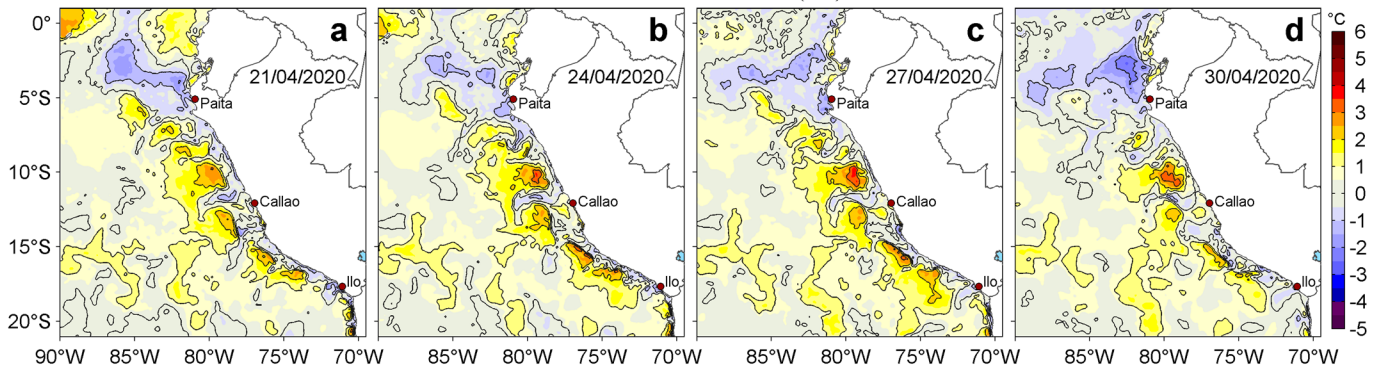
Figura 3. Anomalías de la temperatura superficial del mar (TSM, °C) para los días: a) 21, b) 24, c) 27 y d) 30 de abril de 2020. Las anomalías se calcularon respecto de la climatología para el periodo 2007-2016. Datos: OSTIA-UKMO-L4-GLOB-v2.0 (UK Met Office, 2012; Donlon et al, 2012). Procesamiento: LHF/AFIOF/DGIOCC/IMARPE.
