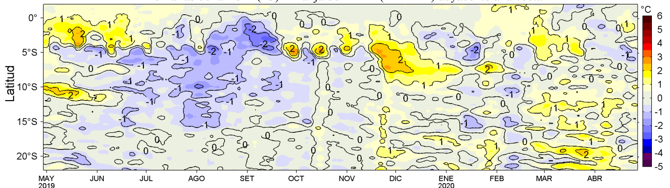
Figura 4. Variación promedio de las anomalías de la temperatura superficial del mar (TSM, °C) para una franja de 60 mn (~111 km) adyacente al litoral peruano para los últimos doce meses al 27 de abril de 2020. Datos: OSTIA-UKMO-L4-GLOB-v2.0 (UK Met. Office, 2012; Donlon et al, 2012) disponible en https://podaac.jpl.nasa.gov/dataset/OSTIA-UKMO-L4-GLOB-v2.0 . Las anomalías se calcularon con respecto al periodo 2007-2016. Procesamiento: LHF/AFIOF/DGIOCC/IMARPE.
