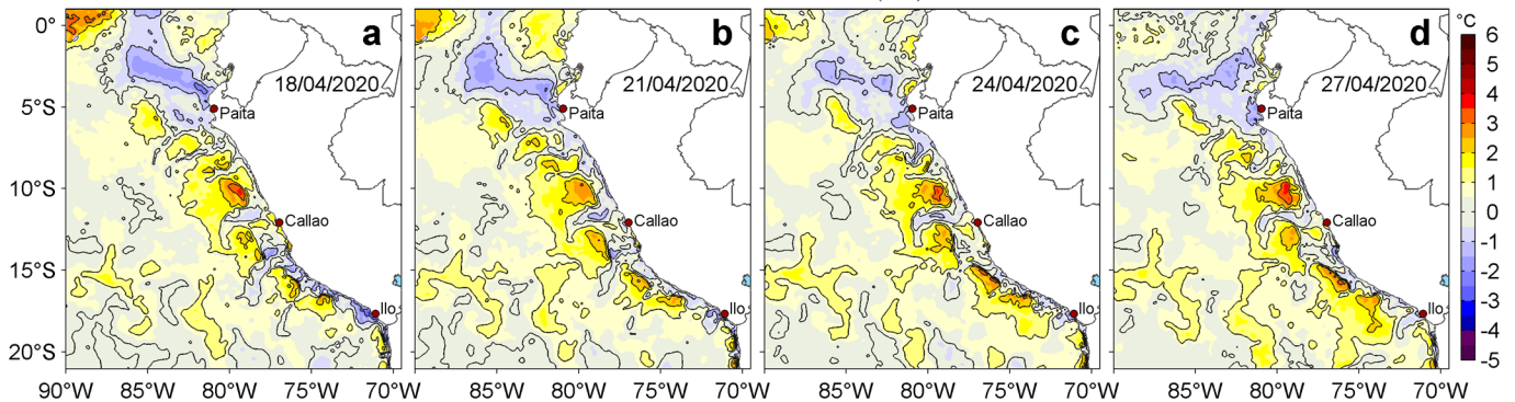
Figura 3. Anomalías de la temperatura superficial del mar (TSM, °C) para los días: a) 18, b) 21, c) 24 y d) 27 de abril de 2020. Las anomalías se calcularon respecto de la climatología para el periodo 2007-2016. Datos: OSTIA-UKMO-L4-GLOB-v2.0 (UK Met Office, 2012; Donlon et al, 2012). Procesamiento: LHF/AFIOF/DGIOCC/IMARPE.
