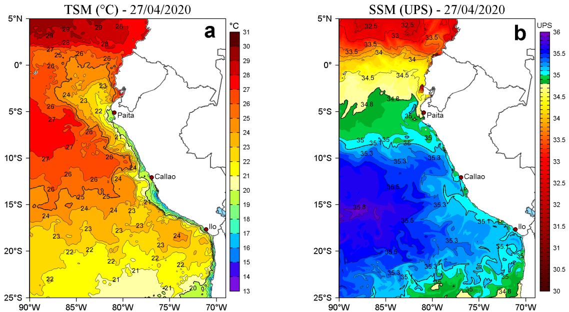
Figura 2. a) Temperatura superficial del mar (TSM, °C) y b) Salinidad superficial del mar (SSM, UPS), para el 27 de abril de 2020. Datos: OSTIA-UKMO-L4-GLOB-v2.0 (UK Met Office, 2012; Donlon et al, 2012) disponible en https://podaac.jpl.nasa.gov/dataset/OSTIA-UKMO-L4-GLOB-v2.0 para (a) y Hybrid Coordinate Ocean Model v. GOFS 3.1 (HYCOM; Halliwell et al., 1998; 2000; Bleck, 2001) para (b). Procesamiento: LHF/AFIOF/DGIOCC/IMARPE.
