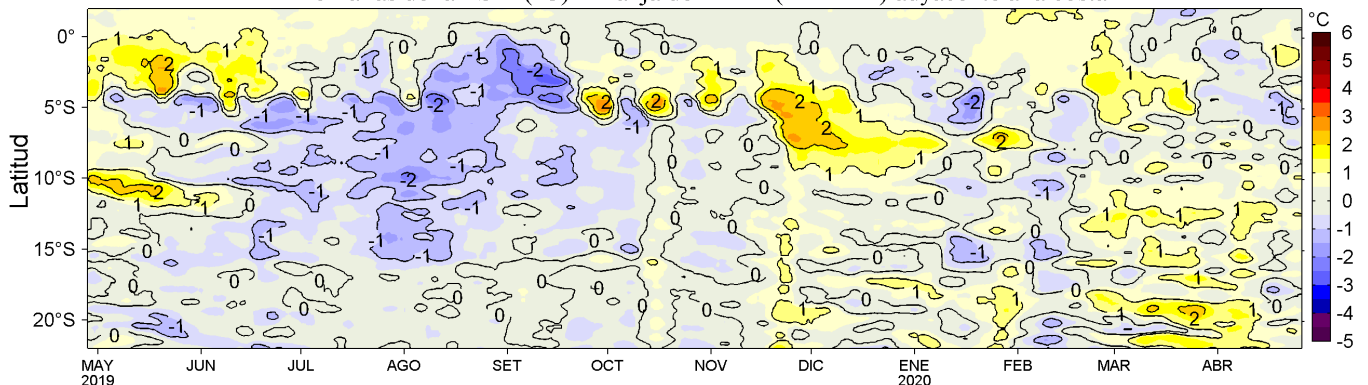
Figura 4. Variación promedio de las anomalías de la temperatura superficial del mar (TSM, °C) para una franja de 60 mn (~111 km) adyacente al litoral peruano para los últimos doce meses al 26 de abril de 2020. Datos: OSTIA-UKMO-L4-GLOB-v2.0 (UK Met. Office, 2012; Donlon et al, 2012) disponible en https://podaac.jpl.nasa.gov/dataset/OSTIA-UKMO-L4-GLOB-v2.0 . Las anomalías se calcularon con respecto al periodo 2007-2016. Procesamiento: LHF/AFIOF/DGIOCC/IMARPE.
