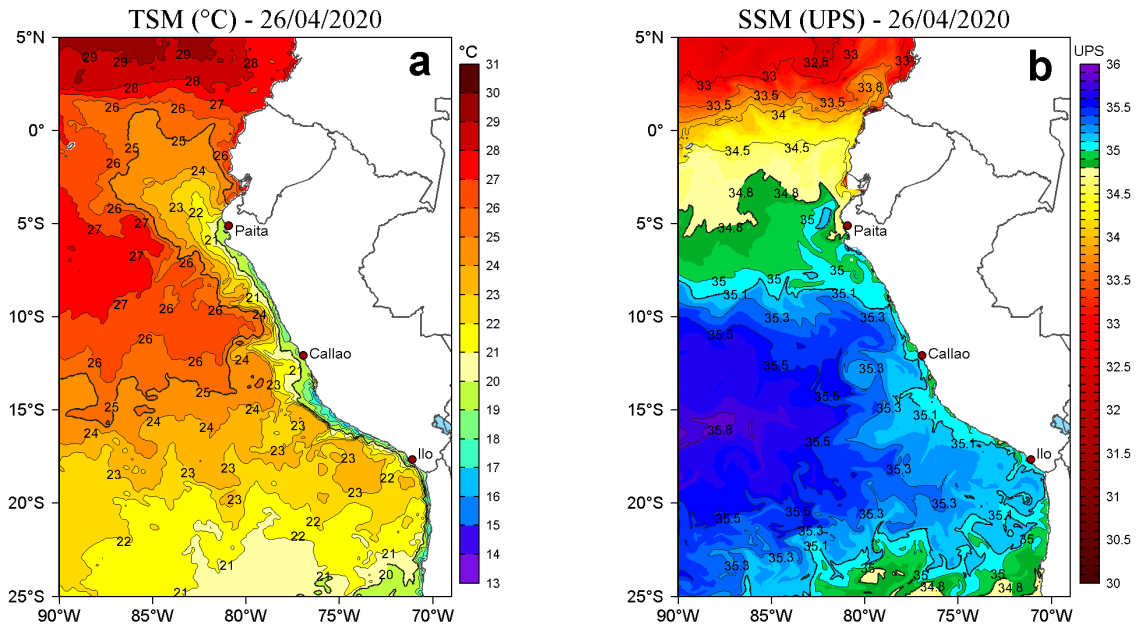
Figura 2. a) Temperatura superficial del mar (TSM, °C) y b) Salinidad superficial del mar (SSM, UPS), para el 26 de abril de 2020. Datos: OSTIA-UKMO-L4-GLOB-v2.0 (UK Met Office, 2012; Donlon et al, 2012) disponible en https://podaac.jpl.nasa.gov/dataset/OSTIA-UKMO-L4-GLOB-v2.0 para (a) y Hybrid Coordinate Ocean Model v. GOFS 3.1 (HYCOM; Halliwell et al., 1998; 2000; Bleck, 2001) para (b). Procesamiento: LHF/AFIOF/DGIOCC/IMARPE.
