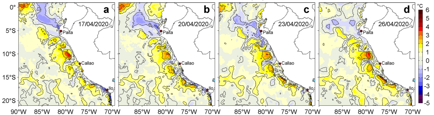
Figura 3. Anomalías de la temperatura superficial del mar (TSM, °C) para los días: a) 17, b) 20, c) 23 y d) 26 de abril de 2020. Las anomalías se calcularon respecto de la climatología para el periodo 2007-2016. Datos: OSTIA-UKMO-L4-GLOB-v2.0 (UK Met Office, 2012; Donlon et al, 2012). Procesamiento: LHF/AFIOF/DGIOCC/IMARPE.
