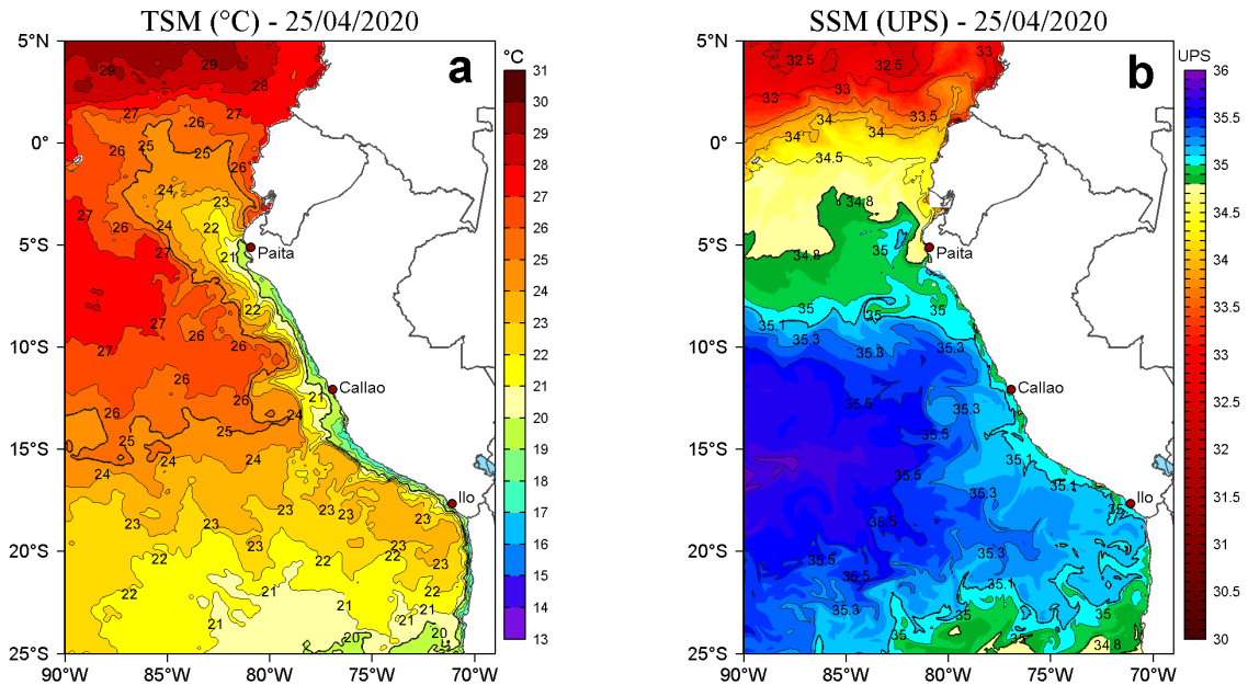
Figura 2. a) Temperatura superficial del mar (TSM, °C) y b) Salinidad superficial del mar (SSM, UPS), para el 25 de abril de 2020. Datos: OSTIA-UKMO-L4-GLOB-v2.0 (UK Met Office, 2012; Donlon et al, 2012) disponible en https://podaac.jpl.nasa.gov/dataset/OSTIA-UKMO-L4-GLOB-v2.0 para (a) y Hybrid Coordinate Ocean Model v. GOFS 3.1 (HYCOM; Halliwell et al., 1998; 2000; Bleck, 2001) para (b). Procesamiento: LHFM/AFIOF/DGIOCC/IMARPE.
