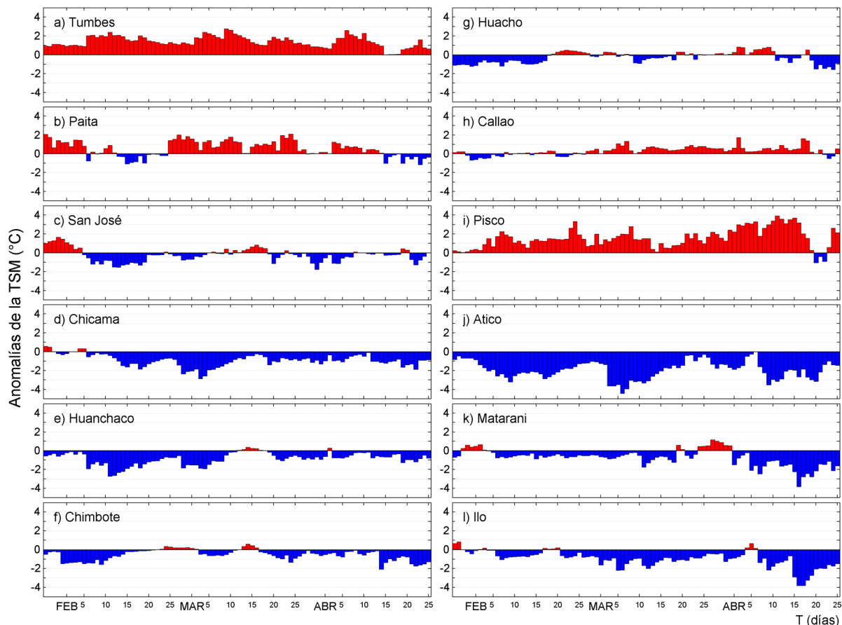
Figura 6. Anomalías de la temperatura superficial del mar (ATSM, °C) satelital durante el último trimestre. La ATSM corresponde a la grilla (~ 6 km) más cercana a la costa frente al muelle de Imapre correspondiente y proviene del producto OSTIA-UKMO-L4-GLOB-v2.0 (UK Met Office, 2012; Donlon et al, 2012) disponible en https://podaac.jpl.nasa.gov/dataset/OSTIA-UKMO-L4-GLOB-v2.0 . Procesamiento: LHF/AFIOF/DGIOCC/IMARPE.
