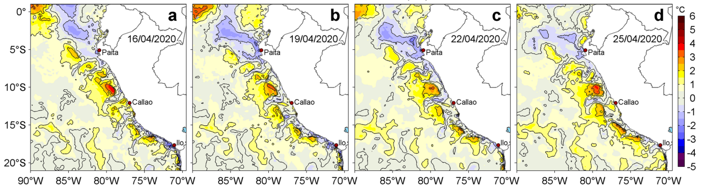
Figura 3. Anomalías de la temperatura superficial del mar (TSM, °C) para los días: a) 16, b) 19, c) 22 y d) 25 de abril de 2020. Las anomalías se calcularon respecto de la climatología para el periodo 2007-2016. Datos: OSTIA-UKMO-L4-GLOB-v2.0 (UK Met Office, 2012; Donlon et al, 2012). Procesamiento: LHFM/AFIOF/DGIOCC/IMARPE.
