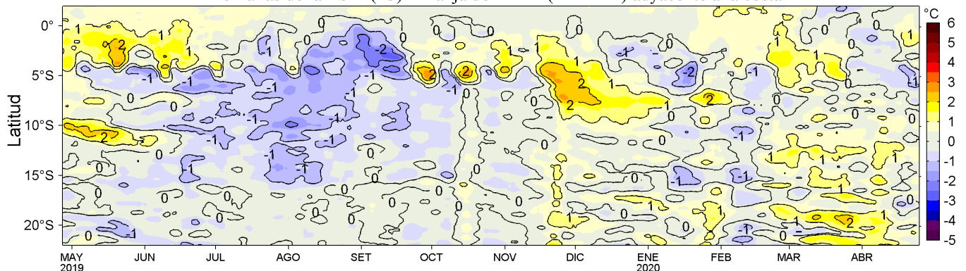
Figura 4. Variación promedio de las anomalías de la temperatura superficial del mar (TSM, °C) para una franja de 60 mn (~111 km) adyacente al litoral peruano para los últimos doce meses al 25 de abril de 2020. Datos: OSTIA-UKMO-L4-GLOB-v2.0 (UK Met. Office, 2012; Donlon et al, 2012) disponible en https://podaac.jpl.nasa.gov/dataset/OSTIA-UKMO-L4-GLOB-v2.0 . Las anomalías se calcularon con respecto al periodo 2007-2016. Procesamiento: LHFM/AFIOF/DGIOCC/IMARPE.
