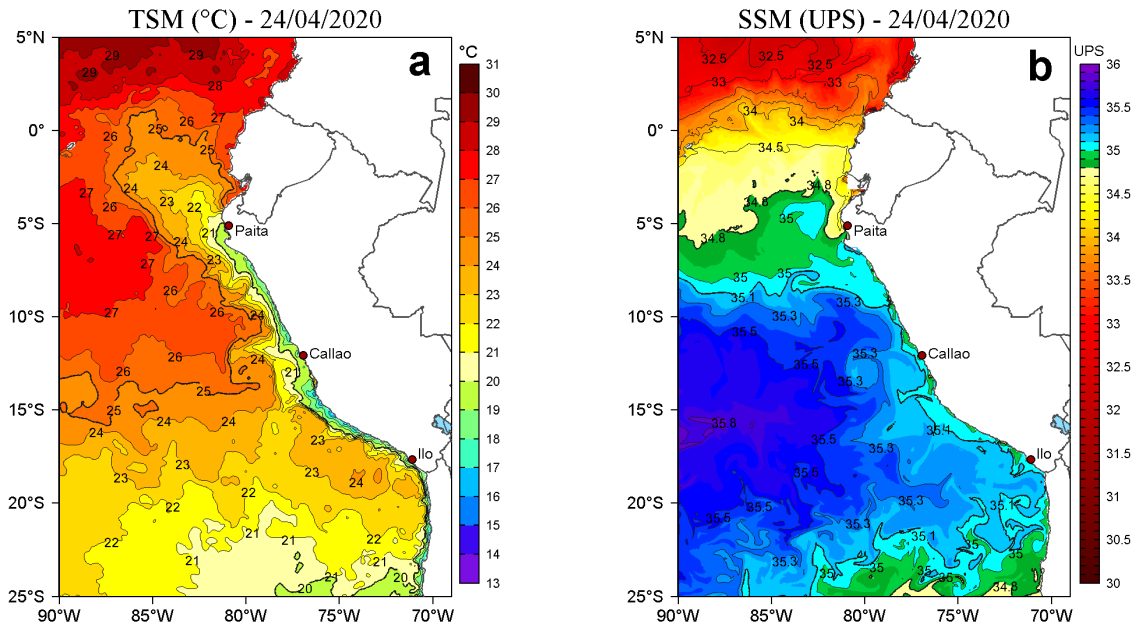
Figura 2. a) Temperatura superficial del mar (TSM, °C) y b) Salinidad superficial del mar (SSM, UPS), para el 24 de abril de 2020. Datos: OSTIA-UKMO-L4-GLOB-v2.0 (UK Met Office, 2012; Donlon et al, 2012) disponible en https://podaac.jpl.nasa.gov/dataset/OSTIA-UKMO-L4-GLOB-v2.0 para (a) y Hybrid Coordinate Ocean Model v. GOFS 3.1 (HYCOM; Halliwell et al., 1998; 2000; Bleck, 2001) para (b). Procesamiento: LHFM/AFIOF/DGIOCC/IMARPE.
