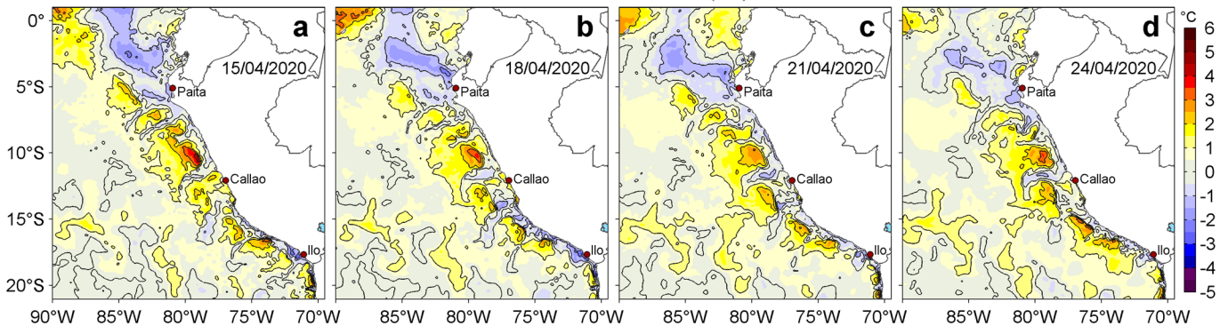
Figura 3. Anomalías de la temperatura superficial del mar (TSM, °C) para los días: a) 15, b) 18, c) 21 y d) 24 de abril de 2020. Las anomalías se calcularon respecto de la climatología para el periodo 2007-2016. Datos: OSTIA-UKMO-L4-GLOB-v2.0 (UK Met Office, 2012; Donlon et al, 2012). Procesamiento: LHFM/AFIOF/DGIOCC/IMARPE.
