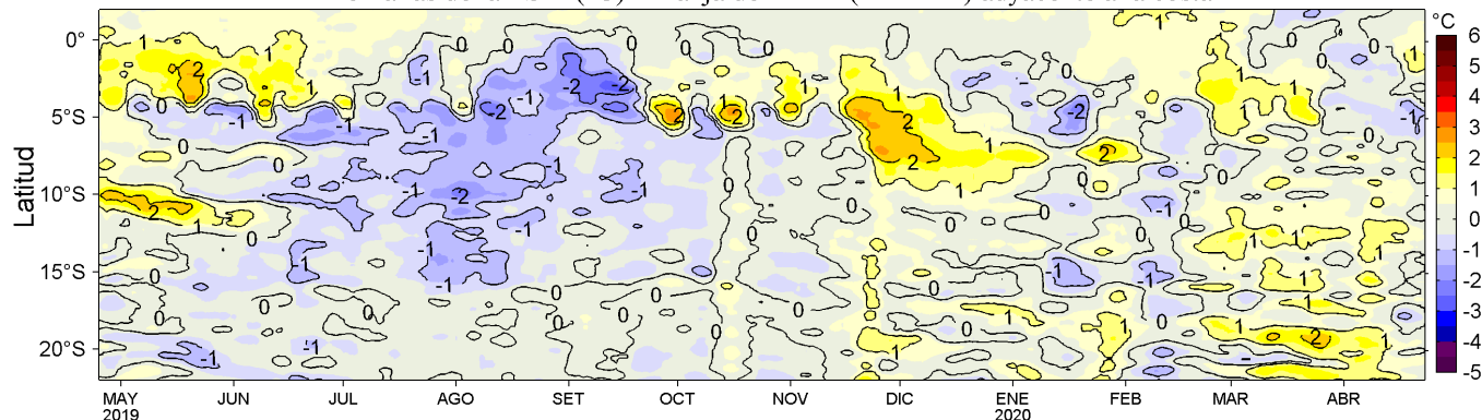
Figura 4. Variación promedio de las anomalías de la temperatura superficial del mar (TSM, °C) para una franja de 60 mn (~111 km) adyacente al litoral peruano para los últimos doce meses al 23 de abril de 2020. Datos: OSTIA-UKMO-L4-GLOB-v2.0 (UK Met. Office, 2012; Donlon et al, 2012) disponible en https://podaac.jpl.nasa.gov/dataset/OSTIA-UKMO-L4-GLOB-v2.0 . Las anomalías se calcularon con respecto al periodo 2007-2016. Procesamiento: LHF/AFIOF/DGIOCC/IMARPE.
