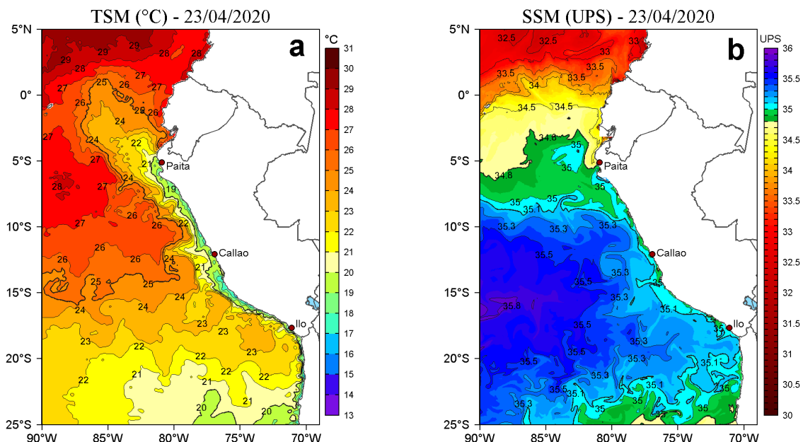
Figura 2. a) Temperatura superficial del mar (TSM, °C) y b) Salinidad superficial del mar (SSM, UPS), para el 23 de abril de 2020. Datos: OSTIA-UKMO-L4-GLOB-v2.0 (UK Met Office, 2012; Donlon et al, 2012) disponible en https://podaac.jpl.nasa.gov/dataset/OSTIA-UKMO-L4-GLOB-v2.0 para (a) y Hybrid Coordinate Ocean Model v. GOFS 3.1 (HYCOM; Halliwell et al., 1998; 2000; Bleck, 2001) para (b). Procesamiento: LHF/AFIOF/DGIOCC/IMARPE.
