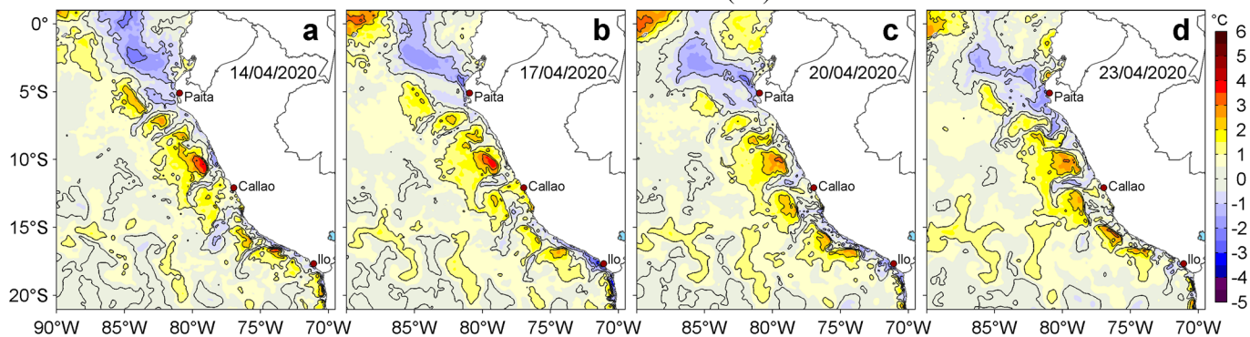
Figura 3. Anomalías de la temperatura superficial del mar (TSM, °C) para los días: a) 14, b) 17, c) 20 y d) 23 de abril de 2020. Las anomalías se calcularon respecto de la climatología para el periodo 2007-2016. Datos: OSTIA-UKMO-L4-GLOB-v2.0 (UK Met Office, 2012; Donlon et al, 2012). Procesamiento: LHF/AFIOF/DGIOCC/IMARPE.
