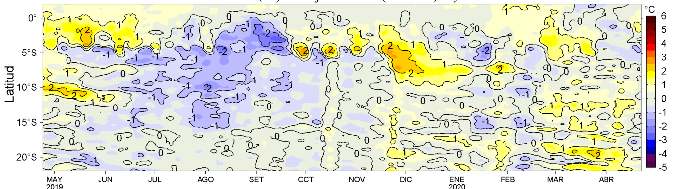
Figura 4. Variación promedio de las anomalías de la temperatura superficial del mar (TSM, °C) para una franja de 60 mn (~111 km) adyacente al litoral peruano para los últimos doce meses al 22 de abril de 2020. Datos: OSTIA-UKMO-L4-GLOB-v2.0 (UK Met. Office, 2012; Donlon et al, 2012) disponible en https://podaac.jpl.nasa.gov/dataset/OSTIA-UKMO-L4-GLOB-v2.0 . Las anomalías se calcularon con respecto al periodo 2007-2016. Procesamiento: LHFH/AFIOF/DGIOCC/IMARPE.
