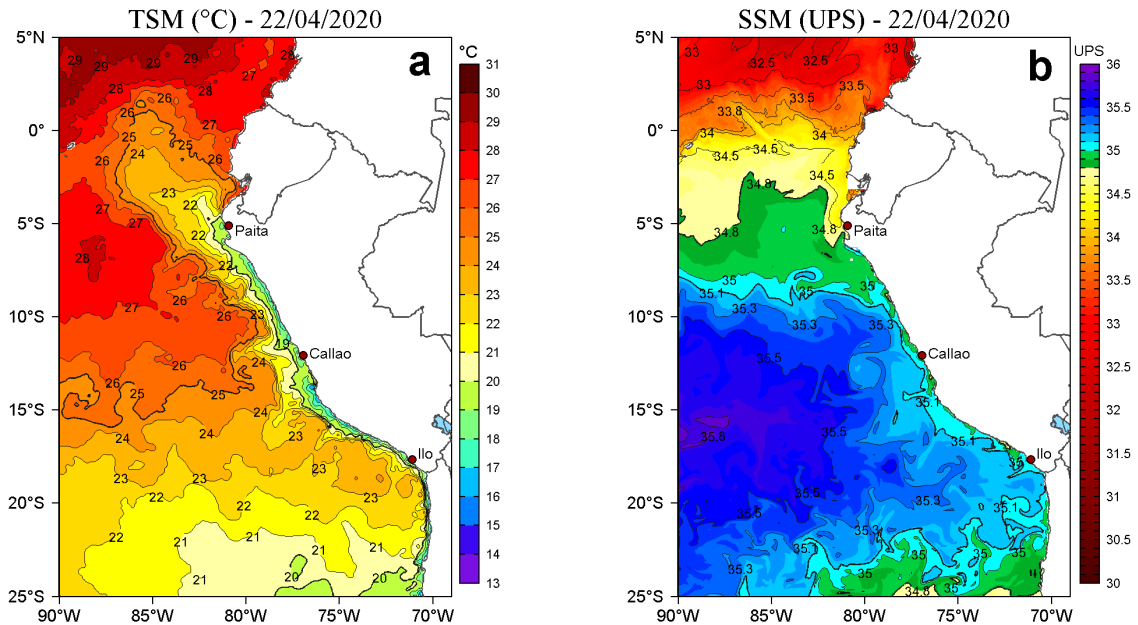
Figura 2. a) Temperatura superficial del mar (TSM, °C) y b) Salinidad superficial del mar (SSM, UPS), para el 22 de abril de 2020. Datos: OSTIA-UKMO-L4-GLOB-v2.0 (UK Met Office, 2012; Donlon et al, 2012) disponible en https://podaac.jpl.nasa.gov/dataset/OSTIA-UKMO-L4-GLOB-v2.0 para (a) y Hybrid Coordinate Ocean Model v. GOFS 3.1 (HYCOM; Halliwell et al., 1998; 2000; Bleck, 2001) para (b). Procesamiento: LHFH/AFIOF/DGIOCC/IMARPE.
