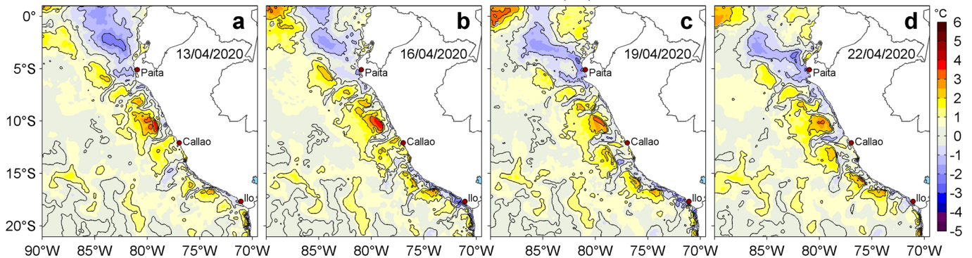
Figura 3. Anomalías de la temperatura superficial del mar (TSM, °C) para los días: a) 13, b) 16, c) 19 y d) 22 de abril de 2020. Las anomalías se calcularon respecto de la climatología para el periodo 2007-2016. Datos: OSTIA-UKMO-L4-GLOB-v2.0 (UK Met Office, 2012; Donlon et al, 2012). Procesamiento: LHFH/AFIOF/DGIOCC/IMARPE.
