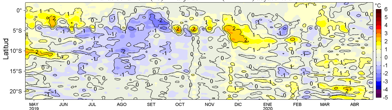
Figura 4. Variación promedio de las anomalías de la temperatura superficial del mar (TSM, °C) para una franja de 60 mn (~111 km) adyacente al litoral peruano para los últimos doce meses al 20 de abril de 2020. Datos: OSTIA-UKMO-L4-GLOB-v2.0 (UK Met. Office, 2012; Donlon et al, 2012) disponible en https://podaac.jpl.nasa.gov/dataset/OSTIA-UKMO-L4-GLOB-v2.0 . Las anomalías se calcularon con respecto al periodo 2007-2016. Procesamiento: LHFM/AFIOF/DGIOCC/IMARPE.
