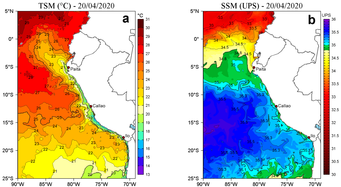
Figura 2. a) Temperatura superficial del mar (TSM, °C) y b) Salinidad superficial del mar (SSM, UPS), para el 20 de abril de 2020. Datos: OSTIA-UKMO-L4-GLOB-v2.0 (UK Met Office, 2012; Donlon et al, 2012) disponible en https://podaac.jpl.nasa.gov/dataset/OSTIA-UKMO-L4-GLOB-v2.0 para (a) y Hybrid Coordinate Ocean Model v. GOFS 3.1 (HYCOM; Halliwell et al., 1998; 2000; Bleck, 2001) para (b). Procesamiento: LHFM/AFIOF/DGIOCC/IMARPE.
