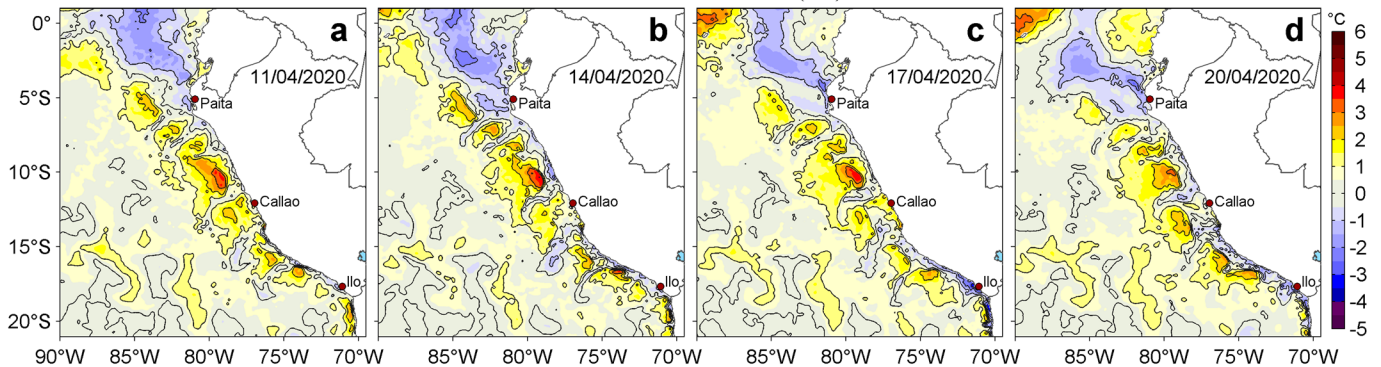
Figura 3. Anomalías de la temperatura superficial del mar (TSM, °C) para los días: a) 11, b) 14, c) 17 y d) 20 de abril de 2020. Las anomalías se calcularon respecto de la climatología para el periodo 2007-2016. Datos: OSTIA-UKMO-L4-GLOB-v2.0 (UK Met Office, 2012; Donlon et al, 2012). Procesamiento: LHFM/AFIOF/DGIOCC/IMARPE.
