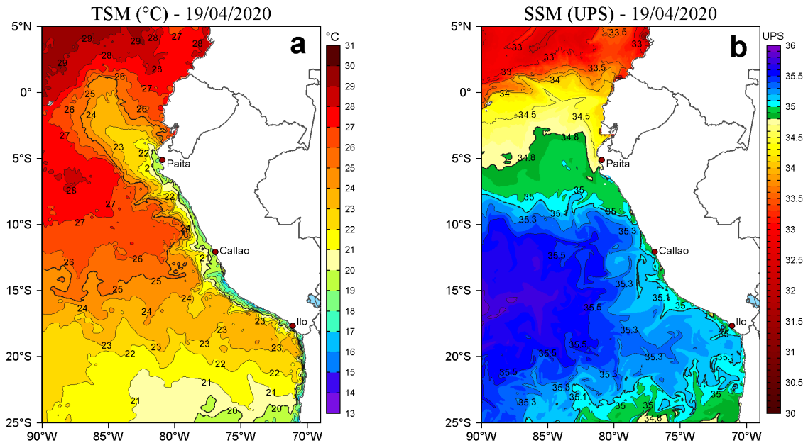
Figura 2. a) Temperatura superficial del mar (TSM, °C) y b) Salinidad superficial del mar (SSM, UPS), para el 19 de abril de 2020. Datos: OSTIA-UKMO-L4-GLOB-v2.0 (UK Met Office, 2012; Donlon et al, 2012) disponible en https://podaac.jpl.nasa.gov/dataset/OSTIA-UKMO-L4-GLOB-v2.0 para (a) y Hybrid Coordinate Ocean Model v. GOFS 3.1 (HYCOM; Halliwell et al., 1998; 2000; Bleck, 2001) para (b). Procesamiento: LHFM/AFIOF/DGIOCC/IMARPE.
