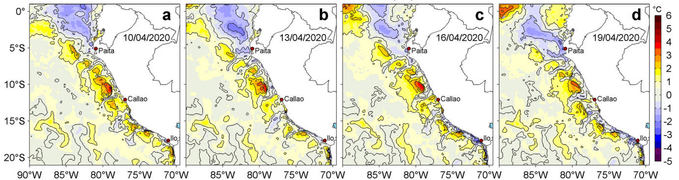
Figura 3. Anomalías de la temperatura superficial del mar (TSM, °C) para los días: a) 10, b) 13, c) 16 y d) 19 de abril de 2020. Las anomalías se calcularon respecto de la climatología para el periodo 2007-2016. Datos: OSTIA-UKMO-L4-GLOB-v2.0 (UK Met Office, 2012; Donlon et al, 2012). Procesamiento: LHFM/AFIOF/DGIOCC/IMARPE.
