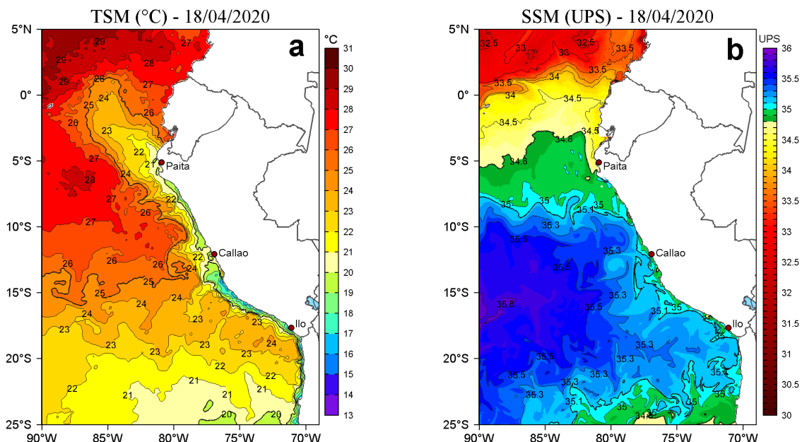
Figura 2. a) Temperatura superficial del mar (TSM, °C) y b) Salinidad superficial del mar (SSM, UPS), para el 18 de abril de 2020. Datos: OSTIA-UKMO-L4-GLOB-v2.0 (UK Met Office, 2012; Donlon et al, 2012) disponible en https://podaac.jpl.nasa.gov/dataset/OSTIA-UKMO-L4-GLOB-v2.0 para (a) y Hybrid Coordinate Ocean Model v. GOFS 3.1 (HYCOM; Halliwell et al., 1998; 2000; Bleck, 2001) para (b). Procesamiento: LHF/AFIOF/DGIOCC/IMARPE.
