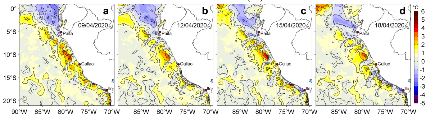
Figura 3. Anomalías de la temperatura superficial del mar (TSM, °C) para los días: a) 09, b) 12, c) 15 y d) 18 de abril de 2020. Las anomalías se calcularon respecto de la climatología para el periodo 2007-2016. Datos: OSTIA-UKMO-L4-GLOB-v2.0 (UK Met Office, 2012; Donlon et al, 2012). Procesamiento: LHF/AFIOF/DGIOCC/IMARPE.
