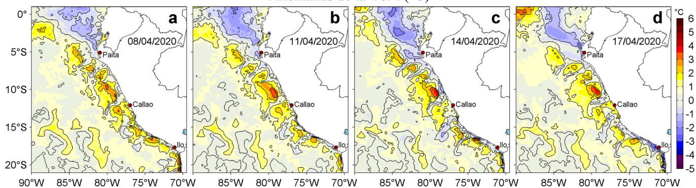
Figura 3. Anomalías de la temperatura superficial del mar (TSM, °C) para los días: a) 08, b) 11, c) 14 y d) 17 de abril de 2020. Las anomalías se calcularon respecto de la climatología para el periodo 2007-2016. Datos: OSTIA-UKMO-L4-GLOB-v2.0 (UK Met Office, 2012; Donlon et al, 2012). Procesamiento: LHFM/AFIOF/DGIOCC/IMARPE.
