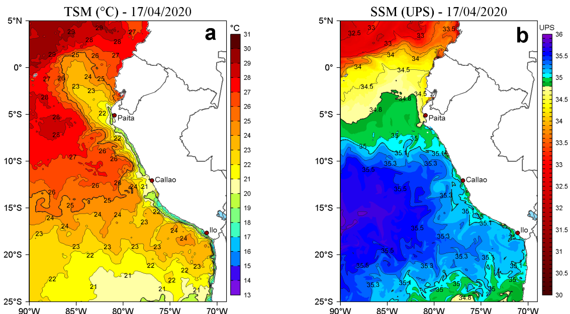
Figura 2. a) Temperatura superficial del mar (TSM, °C) y b) Salinidad superficial del mar (SSM, UPS), para el 17 de abril de 2020. Datos: OSTIA-UKMO-L4-GLOB-v2.0 (UK Met Office, 2012; Donlon et al, 2012) disponible en https://podaac.jpl.nasa.gov/dataset/OSTIA-UKMO-L4-GLOB-v2.0 para (a) y Hybrid Coordinate Ocean Model v. GOFS 3.1 (HYCOM; Halliwell et al., 1998; 2000; Bleck, 2001) para (b). Procesamiento: LHFM/AFIOF/DGIOCC/IMARPE.
