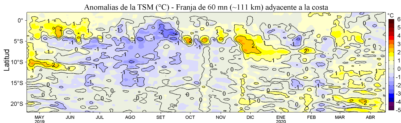
Figura 4. Variación promedio de las anomalías de la temperatura superficial del mar (TSM, °C) para una franja de 60 mn (~111 km) adyacente al litoral peruano para los últimos doce meses al 16 de abril de 2020. Datos: OSTIA-UKMO-L4-GLOB-v2.0 (UK Met. Office, 2012; Donlon et al, 2012) disponible en https://podaac.jpl.nasa.gov/dataset/OSTIA-UKMO-L4-GLOB-v2.0 . Las anomalías se calcularon con respecto al periodo 2007-2016. Procesamiento: LHFM/AFIOF/DGIOCC/IMARPE.
