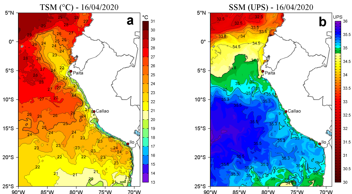
Figura 2. a) Temperatura superficial del mar (TSM, °C) y b) Salinidad superficial del mar (SSM, UPS), para el 16 de abril de 2020. Datos: OSTIA-UKMO-L4-GLOB-v2.0 (UK Met Office, 2012; Donlon et al, 2012) disponible en https://podaac.jpl.nasa.gov/dataset/OSTIA-UKMO-L4-GLOB-v2.0 para (a) y Hybrid Coordinate Ocean Model v. GOFS 3.1 (HYCOM; Halliwell et al., 1998; 2000; Bleck, 2001) para (b). Procesamiento: LHFM/AFIOF/DGIOCC/IMARPE.
