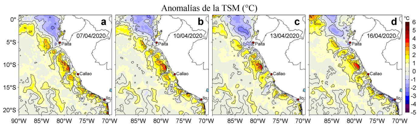
Figura 3. Anomalías de la temperatura superficial del mar (TSM, °C) para los días: a) 07, b) 10, c) 13 y d) 16 de abril de 2020. Las anomalías se calcularon respecto de la climatología para el periodo 2007-2016. Datos: OSTIA-UKMO-L4-GLOB-v2.0 (UK Met Office, 2012; Donlon et al, 2012). Procesamiento: LHFM/AFIOF/DGIOCC/IMARPE.
