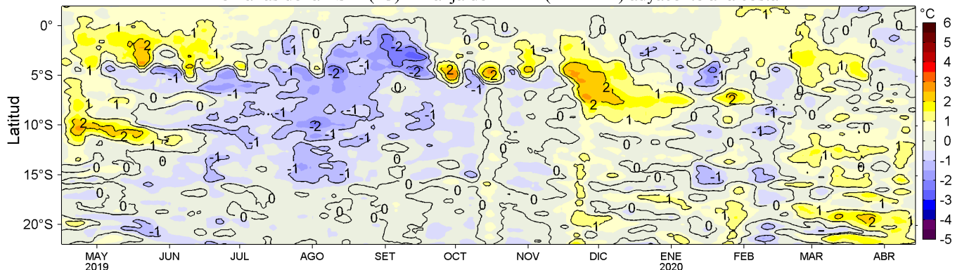
Figura 4. Variación promedio de las anomalías de la temperatura superficial del mar (TSM, °C) para una franja de 60 mn (~111 km) adyacente al litoral peruano para los últimos doce meses al 14 de abril de 2020. Datos: OSTIA-UKMO-L4-GLOB-v2.0 (UK Met. Office, 2012; Donlon et al, 2012) disponible en https://podaac.jpl.nasa.gov/dataset/OSTIA-UKMO-L4-GLOB-v2.0 . Las anomalías se calcularon con respecto al periodo 2007-2016. Procesamiento: LHF/AFIOF/DGIOCC/IMARPE.
