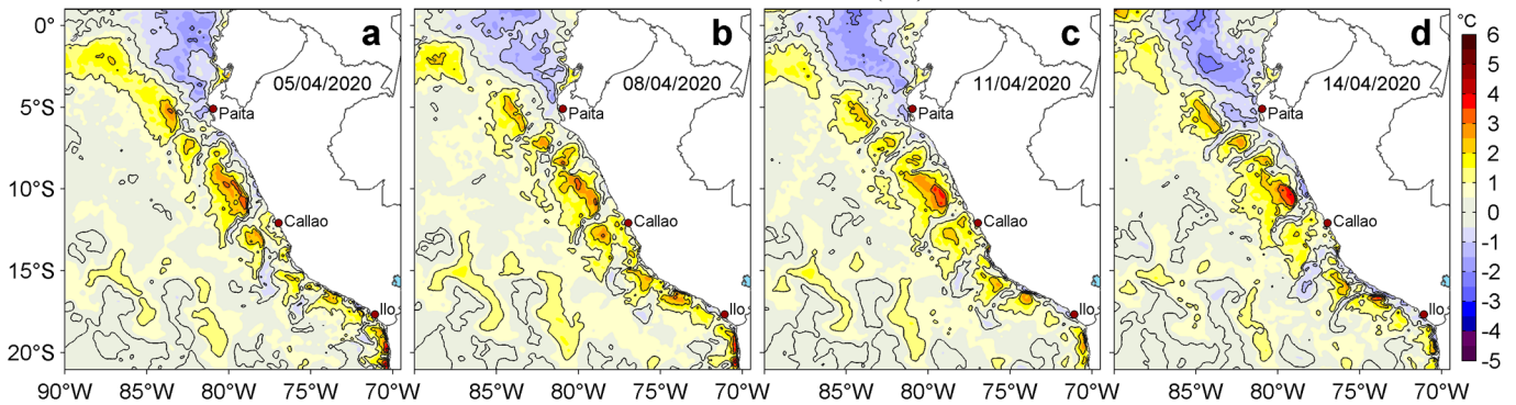
Figura 3. Anomalías de la temperatura superficial del mar (TSM, °C) para los días: a) 05, b) 08, c) 11 y d) 14 de abril de 2020. Las anomalías se calcularon respecto de la climatología para el periodo 2007-2016. Datos: OSTIA-UKMO-L4-GLOB-v2.0 (UK Met Office, 2012; Donlon et al, 2012). Procesamiento: LHF/AFIOF/DGIOCC/IMARPE.
