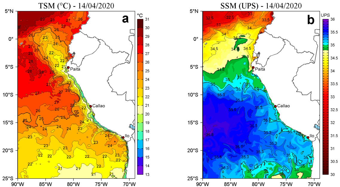
Figura 2. a) Temperatura superficial del mar (TSM, °C) y b) Salinidad superficial del mar (SSM, UPS), para el 14 de abril de 2020. Datos: OSTIA-UKMO-L4-GLOB-v2.0 (UK Met Office, 2012; Donlon et al, 2012) disponible en https://podaac.jpl.nasa.gov/dataset/OSTIA-UKMO-L4-GLOB-v2.0 para (a) y Hybrid Coordinate Ocean Model v. GOFS 3.1 (HYCOM; Halliwell et al., 1998; 2000; Bleck, 2001) para (b). Procesamiento: LHF/AFIOF/DGIOCC/IMARPE.
