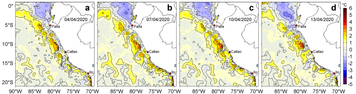
Figura 3. Anomalías de la temperatura superficial del mar (TSM, °C) para los días: a) 04, b) 07, c) 10 y d) 13 de abril de 2020. Las anomalías se calcularon respecto de la climatología para el periodo 2007-2016. Datos: OSTIA-UKMO-L4-GLOB-v2.0 (UK Met Office, 2012; Donlon et al, 2012). Procesamiento: LHF/AFIOF/DGIOCC/IMARPE.
