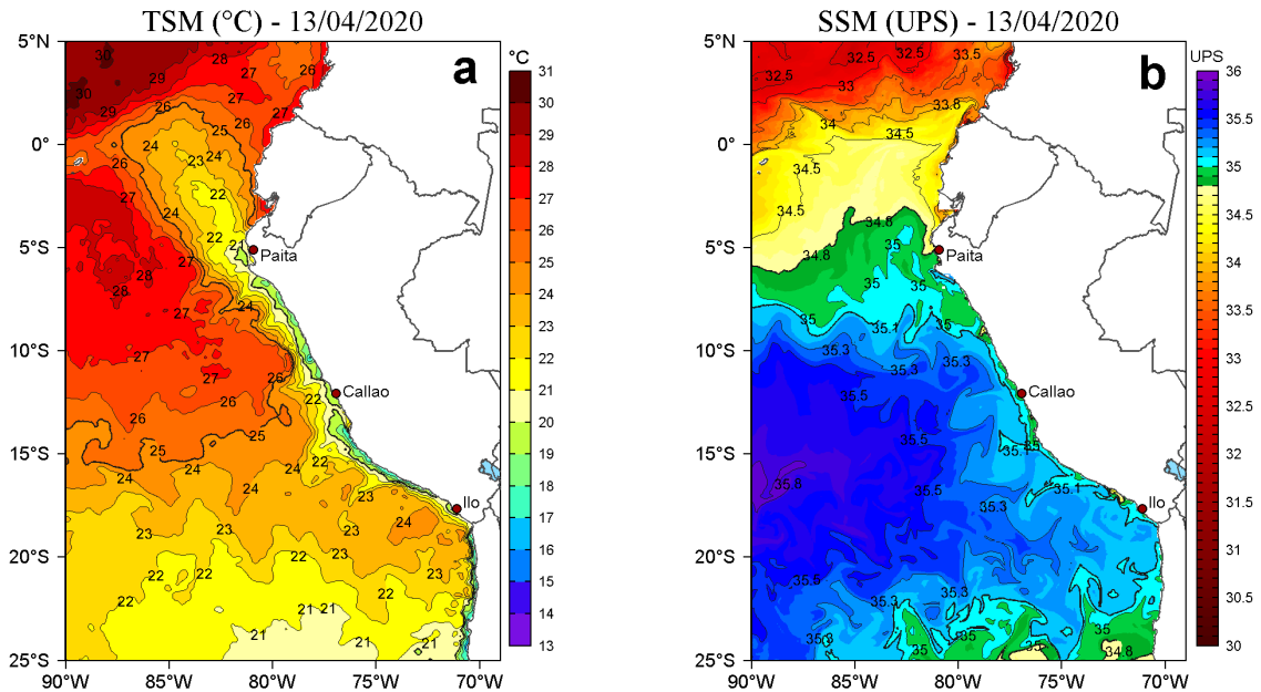
Figura 2. a) Temperatura superficial del mar (TSM, °C) y b) Salinidad superficial del mar (SSM, UPS), para el 13 de abril de 2020. Datos: OSTIA-UKMO-L4-GLOB-v2.0 (UK Met Office, 2012; Donlon et al, 2012) disponible en https://podaac.jpl.nasa.gov/dataset/OSTIA-UKMO-L4-GLOB-v2.0 para (a) y Hybrid Coordinate Ocean Model v. GOFS 3.1 (HYCOM; Halliwell et al., 1998; 2000; Bleck, 2001) para (b). Procesamiento: LHF/AFIOF/DGIOCC/IMARPE.
