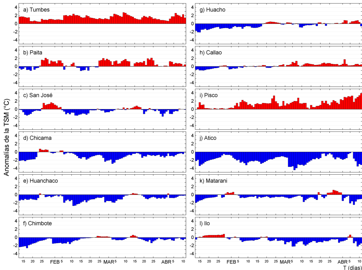
Figura 6. Anomalías de la temperatura superficial del mar (ATSM, °C) satelital durante el último trimestre. La ATSM corresponde a la grilla (~ 6 km) más cercana a la costa frente al muelle de Imape correspondiente y proviene del producto OSTIA-UKMO-L4-GLOB-v2.0 (UK Met Office, 2012; Donlon et al, 2012) disponible en https://podaac.jpl.nasa.gov/dataset/OSTIA-UKMO-L4-GLOB-v2.0 . Procesamiento: LHF/AFIOF/DGIOCC/IMARPE.
