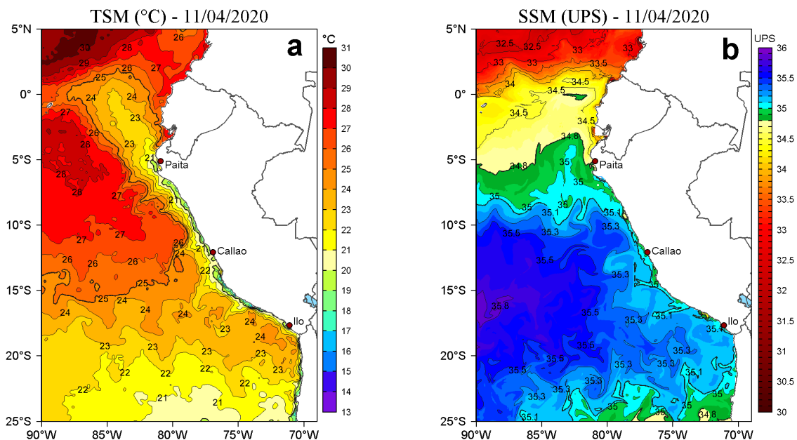
Figura 2. a) Temperatura superficial del mar (TSM, °C) y b) Salinidad superficial del mar (SSM, UPS), para el 11 de abril de 2020. Datos: OSTIA-UKMO-L4-GLOB-v2.0 (UK Met Office, 2012; Donlon et al, 2012) disponible en https://podaac.jpl.nasa.gov/dataset/OSTIA-UKMO-L4-GLOB-v2.0 para (a) y Hybrid Coordinate Ocean Model v. GOFS 3.1 (HYCOM; Halliwell et al., 1998; 2000; Bleck, 2001) para (b). Procesamiento: LHF/AFIOF/DGIOCC/IMARPE.
