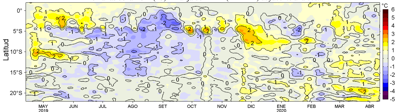
Figura 4. Variación promedio de las anomalías de la temperatura superficial del mar (TSM, °C) para una franja de 60 mn (~111 km) adyacente al litoral peruano para los últimos doce meses al 11 de abril de 2020. Datos: OSTIA-UKMO-L4-GLOB-v2.0 (UK Met. Office, 2012; Donlon et al, 2012) disponible en https://podaac.jpl.nasa.gov/dataset/OSTIA-UKMO-L4-GLOB-v2.0 . Las anomalías se calcularon con respecto al periodo 2007-2016. Procesamiento: LHF/AFIOF/DGIOCC/IMARPE.
