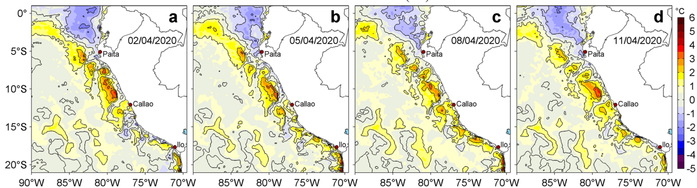
Figura 3. Anomalías de la temperatura superficial del mar (TSM, °C) para los días: a) 02, b) 05, c) 08 y d) 11 de abril de 2020. Las anomalías se calcularon respecto de la climatología para el periodo 2007-2016. Datos: OSTIA-UKMO-L4-GLOB-v2.0 (UK Met Office, 2012; Donlon et al, 2012). Procesamiento: LHF/AFIOF/DGIOCC/IMARPE.
