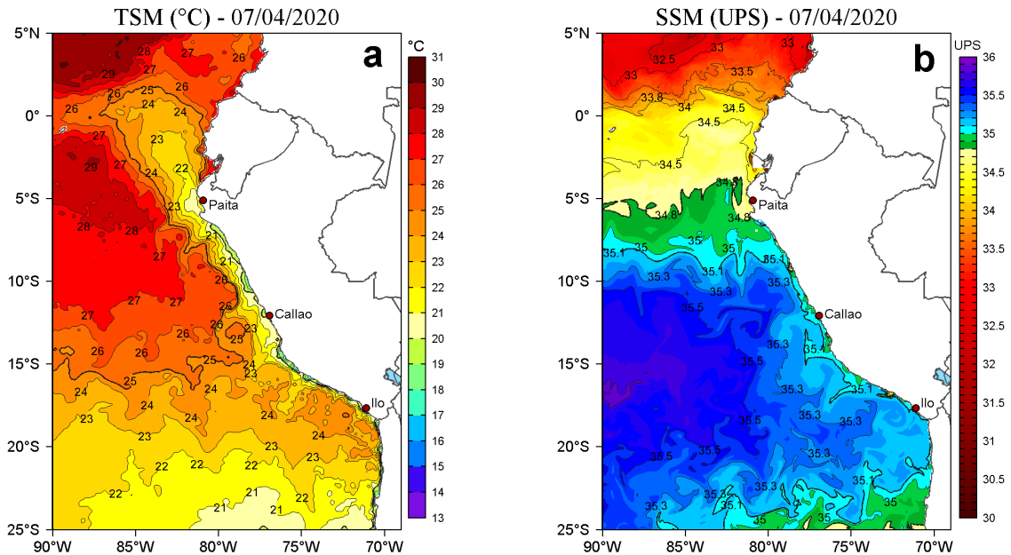
Figura 2. a) Temperatura superficial del mar (TSM, °C) y b) Salinidad superficial del mar (SSM, UPS), para el 07 de abril de 2020. Datos: OSTIA-UKMO-L4-GLOB-v2.0 (UK Met Office, 2012; Donlon et al, 2012) disponible en https://podaac.jpl.nasa.gov/dataset/OSTIA-UKMO-L4-GLOB-v2.0 para (a) y Hybrid Coordinate Ocean Model v. GOFS 3.1 (HYCOM; Halliwell et al., 1998; 2000; Bleck, 2001) para (b). Procesamiento: LHFm/AFIOF/DGIOCC/IMARPE.
