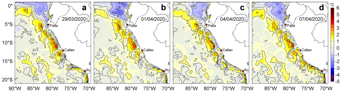
Figura 3. Anomalías de la temperatura superficial del mar (TSM, °C) para los días: a) 29 de marzo, b) 01, c) 04 y d) 07 de abril de 2020. Las anomalías se calcularon respecto de la climatología para el periodo 2007-2016. Datos: OSTIA-UKMO-L4-GLOB-v2.0 (UK Met Office, 2012; Donlon et al, 2012). Procesamiento: LHFm/AFIOF/DGIOCC/IMARPE.
