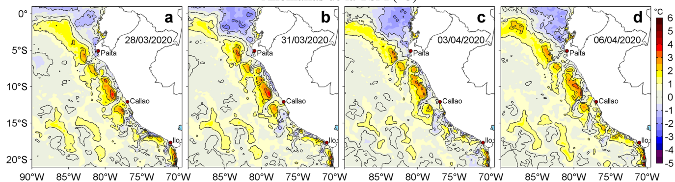
Figura 3. Anomalías de la temperatura superficial del mar (TSM, °C) para los días: a) 28 y b) 31 de marzo, c) 03 y d) 06 de abril de 2020. Las anomalías se calcularon respecto de la climatología para el periodo 2007-2016. Datos: OSTIA-UKMO-L4-GLOB-v2.0 (UK Met Office, 2012; Donlon et al, 2012). Procesamiento: LHFm/AFIOF/DGIOCC/IMARPE.
