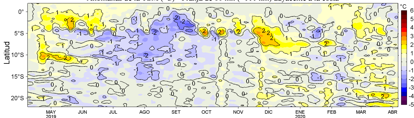
Figura 4. Variación promedio de las anomalías de la temperatura superficial del mar (TSM, °C) para una franja de 60 mn (~111 km) adyacente al litoral peruano para los últimos doce meses al 06 de abril de 2020. Datos: OSTIA-UKMO-L4-GLOB-v2.0 (UK Met. Office, 2012; Donlon et al, 2012) disponible en https://podaac.jpl.nasa.gov/dataset/OSTIA-UKMO-L4-GLOB-v2.0 . Las anomalías se calcularon con respecto al periodo 2007-2016. Procesamiento: LHFm/AFIOF/DGIOCC/IMARPE.
