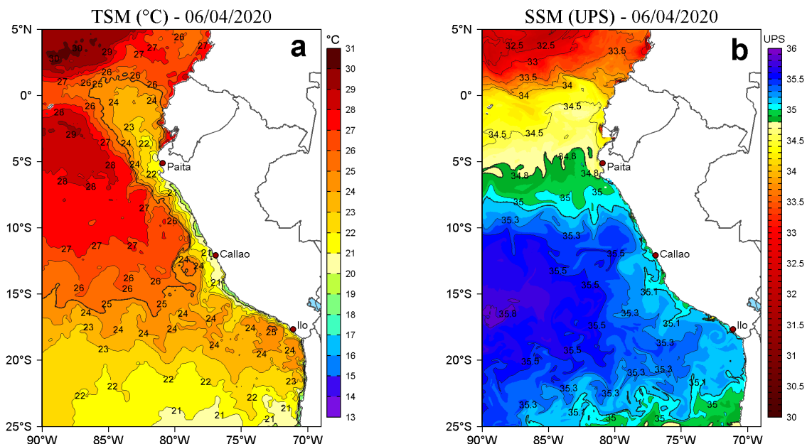
Figura 2. a) Temperatura superficial del mar (TSM, °C) y b) Salinidad superficial del mar (SSM, UPS), para el 06 de abril de 2020. Datos: OSTIA-UKMO-L4-GLOB-v2.0 (UK Met Office, 2012; Donlon et al, 2012) disponible en https://podaac.jpl.nasa.gov/dataset/OSTIA-UKMO-L4-GLOB-v2.0 para (a) y Hybrid Coordinate Ocean Model v. GOFS 3.1 (HYCOM; Halliwell et al., 1998; 2000; Bleck, 2001) para (b). Procesamiento: LHFm/AFIOF/DGIOCC/IMARPE.
