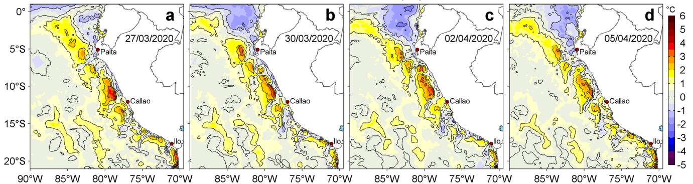
Figura 3. Anomalías de la temperatura superficial del mar (TSM, °C) para los días: a) 27 y b) 30 de marzo, c) 02 y d) 05 de abril de 2020. Las anomalías se calcularon respecto de la climatología para el periodo 2007-2016. Datos: OSTIA-UKMO-L4-GLOB-v2.0 (UK Met Office, 2012; Donlon et al, 2012). Procesamiento: LHFm/AFIOF/DGIOCC/IMARPE.
