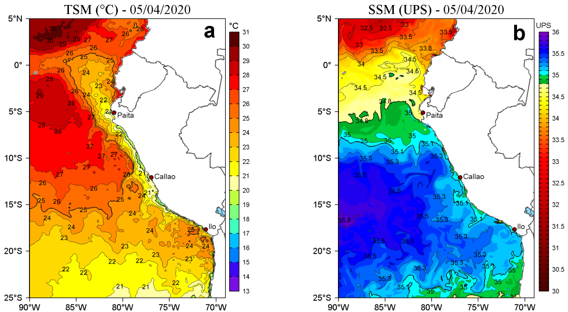
Figura 2. a) Temperatura superficial del mar (TSM, °C) y b) Salinidad superficial del mar (SSM, UPS), para el 05 de abril de 2020. Datos: OSTIA-UKMO-L4-GLOB-v2.0 (UK Met Office, 2012; Donlon et al, 2012) disponible en https://podaac.jpl.nasa.gov/dataset/OSTIA-UKMO-L4-GLOB-v2.0 para (a) y Hybrid Coordinate Ocean Model v. GOFS 3.1 (HYCOM; Halliwell et al., 1998; 2000; Bleck, 2001) para (b). Procesamiento: LHFm/AFIOF/DGIOCC/IMARPE.
