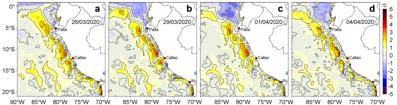
Figura 3. Anomalías de la temperatura superficial del mar (TSM, °C) para los días: a) 26 y b) 29 de marzo, c) 01 y d) 04 de abril de 2020. Las anomalías se calcularon respecto de la climatología para el periodo 2007-2016. Datos: OSTIA-UKMO-L4-GLOB-v2.0 (UK Met Office, 2012; Donlon et al, 2012). Procesamiento: LHFm/AFIOF/DGIOCC/IMARPE.
