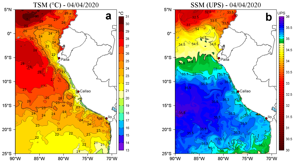
Figura 2. a) Temperatura superficial del mar (TSM, °C) y b) Salinidad superficial del mar (SSM, UPS), para el 04 de abril de 2020. Datos: OSTIA-UKMO-L4-GLOB-v2.0 (UK Met Office, 2012; Donlon et al, 2012) disponible en https://podaac.jpl.nasa.gov/dataset/OSTIA-UKMO-L4-GLOB-v2.0 para (a) y Hybrid Coordinate Ocean Model v. GOFS 3.1 (HYCOM; Halliwell et al., 1998; 2000; Bleck, 2001) para (b). Procesamiento: LHFm/AFIOF/DGIOCC/IMARPE.
