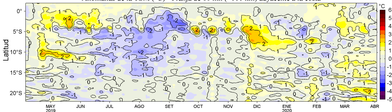
Figura 4. Variación promedio de las anomalías de la temperatura superficial del mar (TSM, °C) para una franja de 60 mn (~111 km) adyacente al litoral peruano para los últimos doce meses al 03 de abril de 2020. Datos: OSTIA-UKMO-L4-GLOB-v2.0 (UK Met. Office, 2012; Donlon et al, 2012) disponible en https://podaac.jpl.nasa.gov/dataset/OSTIA-UKMO-L4-GLOB-v2.0 . Las anomalías se calcularon con respecto al periodo 2007-2016. Procesamiento: LHFm/AFIOF/DGIOCC/IMARPE.
