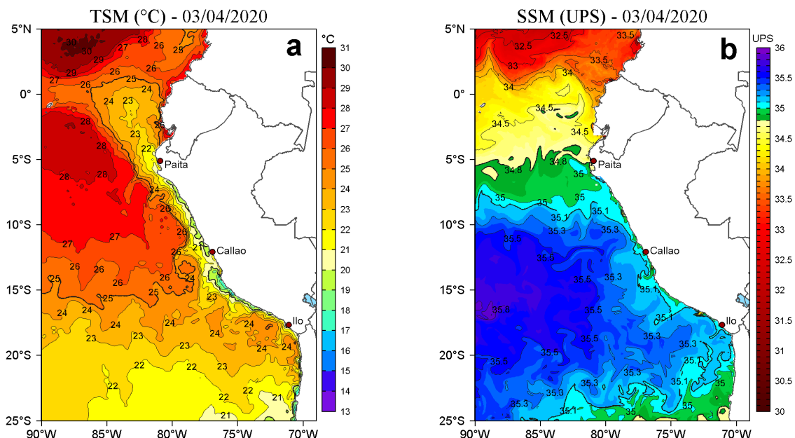
Figura 2. a) Temperatura superficial del mar (TSM, °C) y b) Salinidad superficial del mar (SSM, UPS), para el 03 de abril de 2020. Datos: OSTIA-UKMO-L4-GLOB-v2.0 (UK Met Office, 2012; Donlon et al, 2012) disponible en https://podaac.jpl.nasa.gov/dataset/OSTIA-UKMO-L4-GLOB-v2.0 para (a) y Hybrid Coordinate Ocean Model v. GOFS 3.1 (HYCOM; Halliwell et al., 1998; 2000; Bleck, 2001) para (b). Procesamiento: LHFm/AFIOF/DGIOCC/IMARPE.
