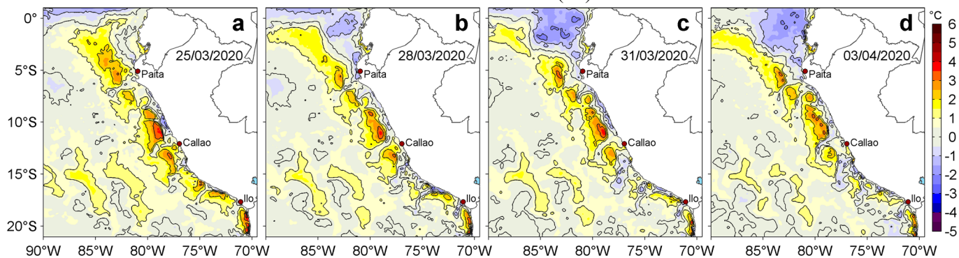
Figura 3. Anomalías de la temperatura superficial del mar (TSM, °C) para los días: a) 25, b) 28 y c) 31 de marzo y d) 03 de abril de 2020. Las anomalías se calcularon respecto de la climatología para el periodo 2007-2016. Datos: OSTIA-UKMO-L4-GLOB-v2.0 (UK Met Office, 2012; Donlon et al, 2012). Procesamiento: LHFm/AFIOF/DGIOCC/IMARPE.
