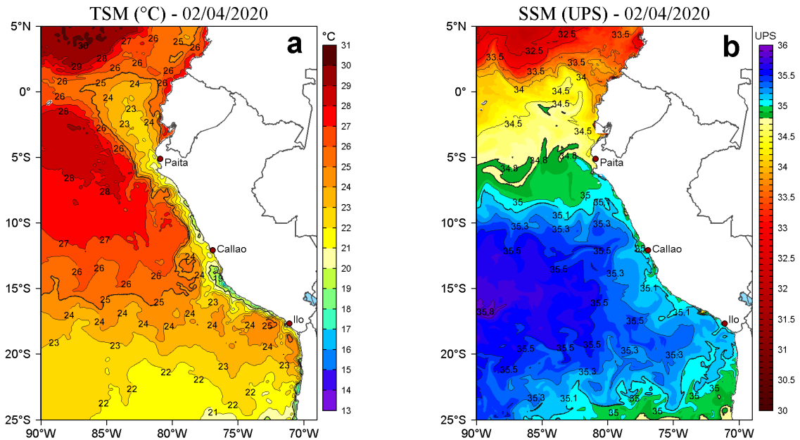
Figura 2. a) Temperatura superficial del mar (TSM, °C) y b) Salinidad superficial del mar (SSM, UPS), para el 02 de abril de 2020. Datos: OSTIA-UKMO-L4-GLOB-v2.0 (UK Met Office, 2012; Donlon et al, 2012) disponible en https://podaac.jpl.nasa.gov/dataset/OSTIA-UKMO-L4-GLOB-v2.0 para (a) y Hybrid Coordinate Ocean Model v. GOFS 3.1 (HYCOM; Halliwell et al., 1998; 2000; Bleck, 2001) para (b). Procesamiento: LHFm/AFIOF/DGIOCC/IMARPE.
