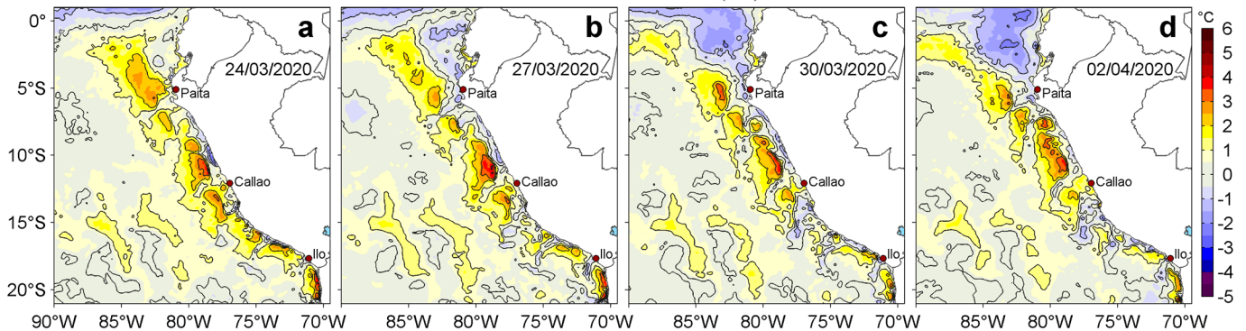
Figura 3. Anomalías de la temperatura superficial del mar (TSM, °C) para los días: a) 24, b) 27 y c) 30 de marzo y d) 02 de abril de 2020. Las anomalías se calcularon respecto de la climatología para el periodo 2007-2016. Datos: OSTIA-UKMO-L4-GLOB-v2.0 (UK Met Office, 2012; Donlon et al, 2012). Procesamiento: LHFm/AFIOF/DGIOCC/IMARPE.
