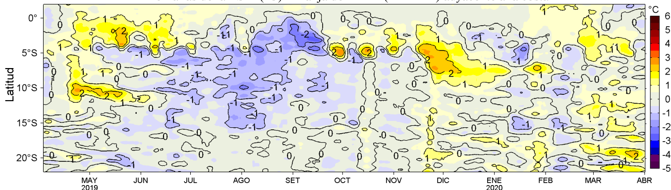
Figura 4. Variación promedio de las anomalías de la temperatura superficial del mar (TSM, °C) para una franja de 60 mn (~111 km) adyacente al litoral peruano para los últimos doce meses al 01 de abril de 2020. Datos: OSTIA-UKMO-L4-GLOB-v2.0 (UK Met. Office, 2012; Donlon et al, 2012) disponible en https://podaac.jpl.nasa.gov/dataset/OSTIA-UKMO-L4-GLOB-v2.0 . Las anomalías se calcularon con respecto al periodo 2007-2016. Procesamiento: LHFm/AFIOF/DGIOCC/IMARPE.
