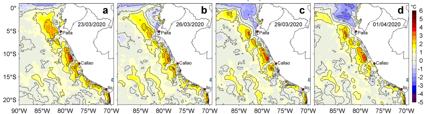
Figura 3. Anomalías de la temperatura superficial del mar (TSM, °C) para los días: a) 23, b) 26 y c) 29 de marzo y d) 01 de abril de 2020. Las anomalías se calcularon respecto de la climatología para el periodo 2007-2016. Datos: OSTIA-UKMO-L4-GLOB-v2.0 (UK Met Office, 2012; Donlon et al, 2012). Procesamiento: LHFm/AFIOF/DGIOCC/IMARPE.
