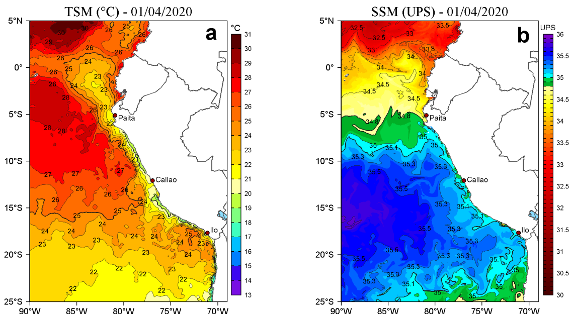
Figura 2. a) Temperatura superficial del mar (TSM, °C) y b) Salinidad superficial del mar (SSM, UPS), para el 01 de abril de 2020. Datos: OSTIA-UKMO-L4-GLOB-v2.0 (UK Met Office, 2012; Donlon et al, 2012) disponible en https://podaac.jpl.nasa.gov/dataset/OSTIA-UKMO-L4-GLOB-v2.0 para (a) y Hybrid Coordinate Ocean Model v. GOFS 3.1 (HYCOM; Halliwell et al., 1998; 2000; Bleck, 2001) para (b). Procesamiento: LHFm/AFIOF/DGIOCC/IMARPE.
