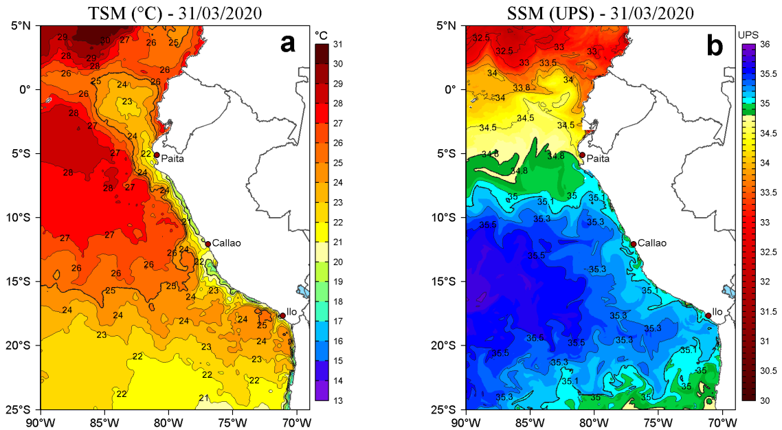
Figura 2. a) Temperatura superficial del mar (TSM, °C) y b) Salinidad superficial del mar (SSM, UPS), para el 31 de marzo de 2020. Datos: OSTIA-UKMO-L4-GLOB-v2.0 (UK Met Office, 2012; Donlon et al, 2012) disponible en https://podaac.jpl.nasa.gov/dataset/OSTIA-UKMO-L4-GLOB-v2.0 para (a) y Hybrid Coordinate Ocean Model v. GOF3 3.1 (HYCOM; Halliwell et al., 1998; 2000; Bleck, 2001) para (b). Procesamiento: LHF/AFIOF/DGIOCC/IMARPE.
