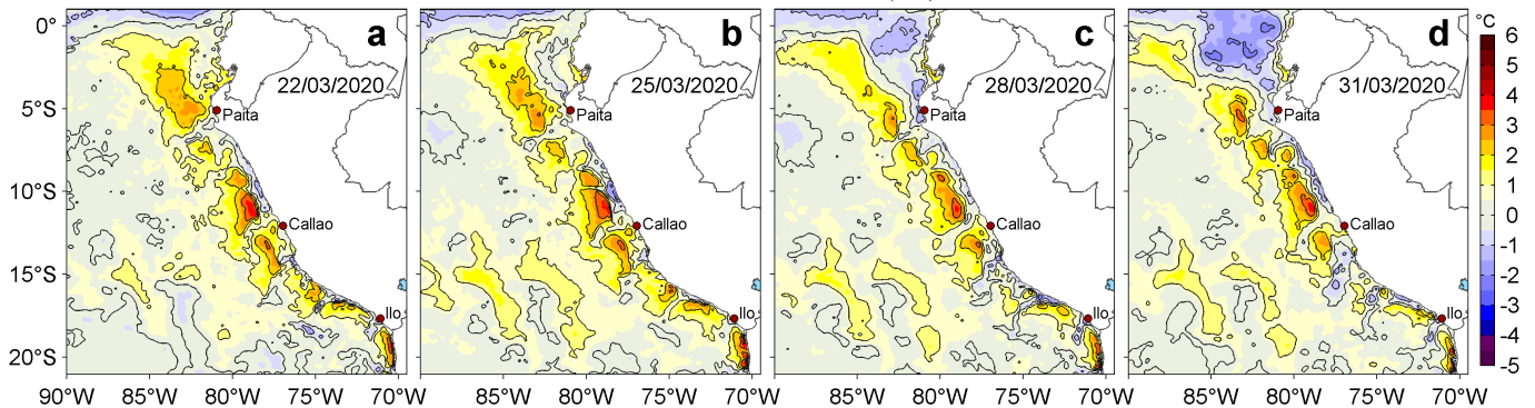
Figura 3. Anomalías de la temperatura superficial del mar (TSM, °C) para los días: a) 22, b) 25, c) 28 y d) 31 de marzo de 2020. Las anomalías se calcularon respecto de la climatología para el periodo 2007-2016. Datos: OSTIA-UKMO-L4-GLOB-v2.0 (UK Met Office, 2012; Donlon et al, 2012). Procesamiento: LHF/AFIOF/DGIOCC/IMARPE.
