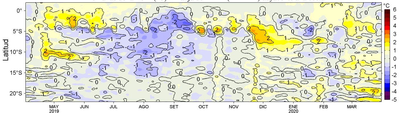
Figura 4. Variación promedio de las anomalías de la temperatura superficial del mar (TSM, °C) para una franja de 60 mn (~111 km) adyacente al litoral peruano para los últimos doce meses al 31 de marzo de 2020. Datos: OSTIA-UKMO-L4-GLOB-v2.0 (UK Met. Office, 2012; Donlon et al, 2012) disponible en https://podaac.jpl.nasa.gov/dataset/OSTIA-UKMO-L4-GLOB-v2.0 . Las anomalías se calcularon con respecto al periodo 2007-2016. Procesamiento: LHF/AFIOF/DGIOCC/IMARPE.
