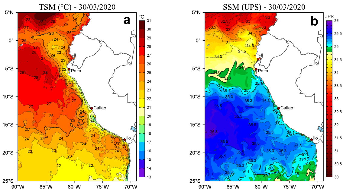
Figura 2. a) Temperatura superficial del mar (TSM, °C) y b) Salinidad superficial del mar (SSM, UPS), para el 30 de marzo de 2020. Datos: OSTIA-UKMO-L4-GLOB-v2.0 (UK Met Office, 2012; Donlon et al, 2012) disponible en https://podaac.jpl.nasa.gov/dataset/OSTIA-UKMO-L4-GLOB-v2.0 para (a) y Hybrid Coordinate Ocean Model v. GOFS 3.1 (HYCOM; Halliwell et al., 1998; 2000; Bleck, 2001) para (b). Procesamiento: LHF/AFIOF/DGIOCC/IMARPE.
