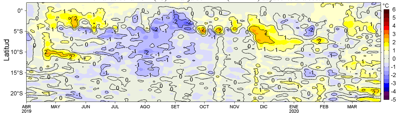
Figura 4. Variación promedio de las anomalías de la temperatura superficial del mar (TSM, °C) para una franja de 60 mn (~111 km) adyacente al litoral peruano para los últimos doce meses al 30 de marzo de 2020. Datos: OSTIA-UKMO-L4-GLOB-v2.0 (UK Met. Office, 2012; Donlon et al, 2012) disponible en https://podaac.jpl.nasa.gov/dataset/OSTIA-UKMO-L4-GLOB-v2.0 . Las anomalías se calcularon con respecto al periodo 2007-2016. Procesamiento: LHF/AFIOF/DGIOCC/IMARPE.
