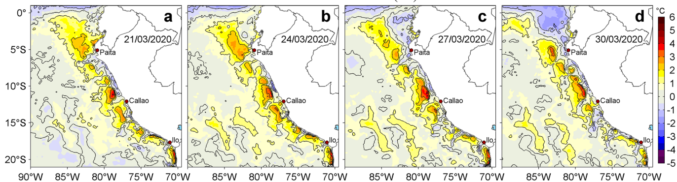
Figura 3. Anomalías de la temperatura superficial del mar (TSM, °C) para los días: a) 21, b) 24, c) 27 y d) 30 de marzo de 2020. Las anomalías se calcularon respecto de la climatología para el periodo 2007-2016. Datos: OSTIA-UKMO-L4-GLOB-v2.0 (UK Met Office, 2012; Donlon et al, 2012). Procesamiento: LHF/AFIOF/DGIOCC/IMARPE.
