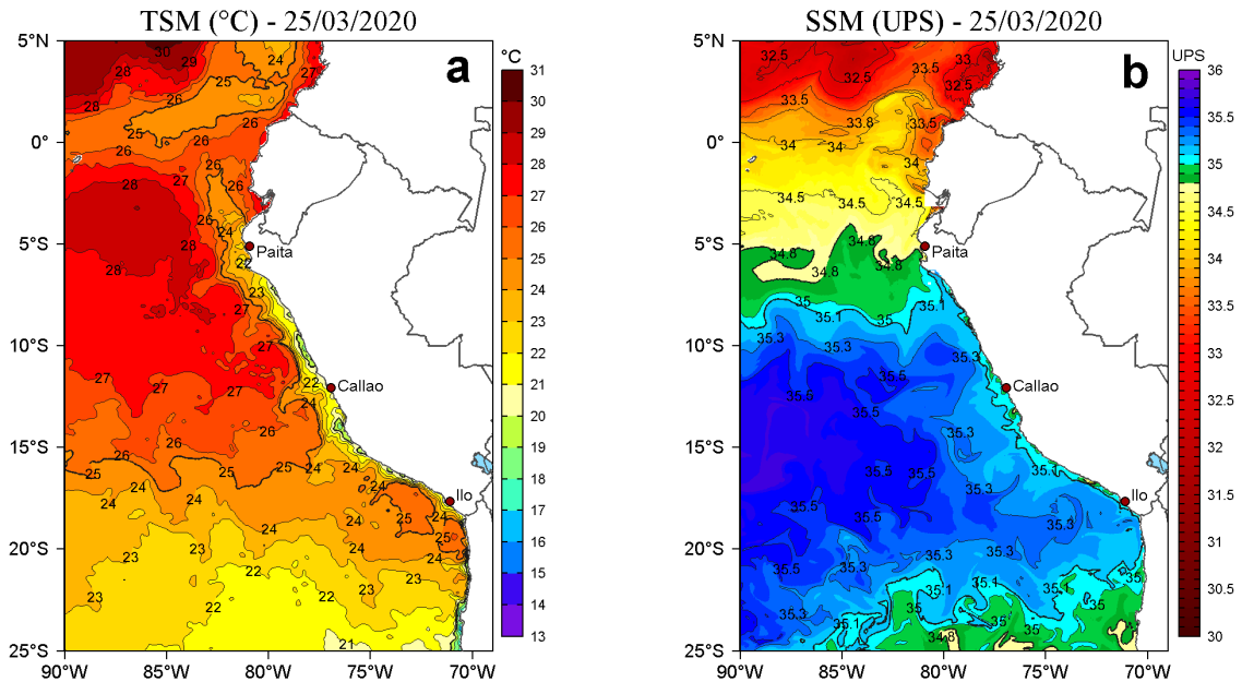
Figura 2. a) Temperatura superficial del mar (TSM, °C) y b) Salinidad superficial del mar (SSM, UPS), para el 25 de marzo de 2020. Datos: OSTIA-UKMO-L4-GLOB-v2.0 (UK Met Office, 2012; Donlon et al, 2012) disponible en https://podaac.jpl.nasa.gov/dataset/OSTIA-UKMO-L4-GLOB-v2.0 para (a) y Hybrid Coordinate Ocean Model v. GOFS 3.1 (HYCOM; Halliwell et al., 1998; 2000; Bleck, 2001) para (b). Procesamiento: LHFm/AFIOF/DGIOCC/IMARPE.
