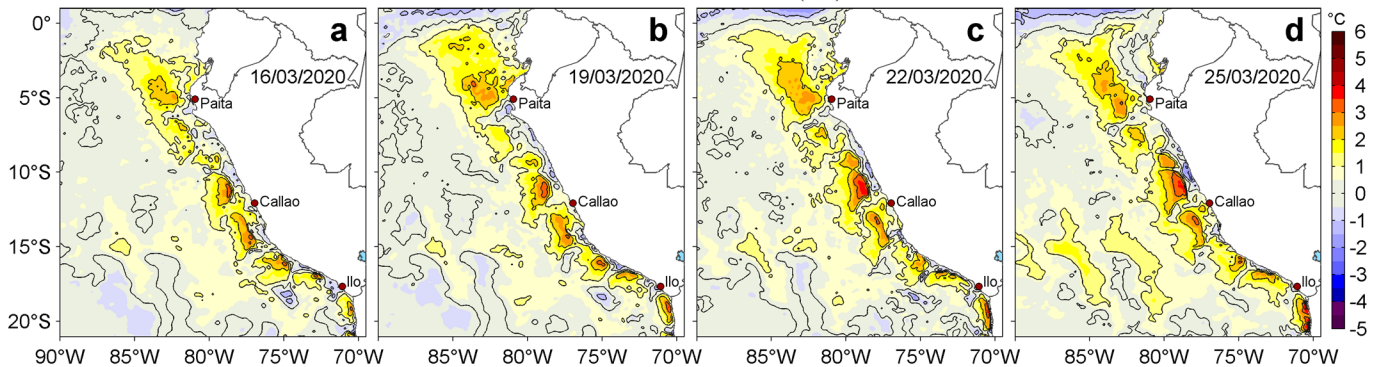
Figura 3. Anomalías de la temperatura superficial del mar (TSM, °C) para los días: a) 16, b) 19, c) 22 y d) 25 de marzo de 2020. Las anomalías se calcularon respecto de la climatología para el periodo 2007-2016. Datos: OSTIA-UKMO-L4-GLOB-v2.0 (UK Met Office, 2012; Donlon et al, 2012). Procesamiento: LHFm/AFIOF/DGIOCC/IMARPE.
