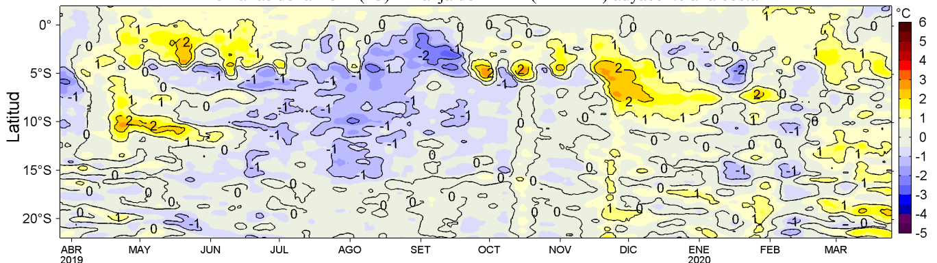
Figura 4. Variación promedio de las anomalías de la temperatura superficial del mar (TSM, °C) para una franja de 60 mn (~111 km) adyacente al litoral peruano para los últimos doce meses al 25 de marzo de 2020. Datos: OSTIA-UKMO-L4-GLOB-v2.0 (UK Met. Office, 2012; Donlon et al, 2012) disponible en https://podaac.jpl.nasa.gov/dataset/OSTIA-UKMO-L4-GLOB-v2.0 . Las anomalías se calcularon con respecto al periodo 2007-2016. Procesamiento: LHFm/AFIOF/DGIOCC/IMARPE.
