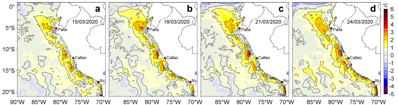
Figura 3. Anomalías de la temperatura superficial del mar (TSM, °C) para los días: a) 15, b) 18, c) 21 y d) 24 de marzo de 2020. Las anomalías se calcularon respecto de la climatología para el periodo 2007-2016. Datos: OSTIA-UKMO-L4-GLOB-v2.0 (UK Met Office, 2012; Donlon et al, 2012). Procesamiento: LHF/AFIOF/DGIOCC/IMARPE.
