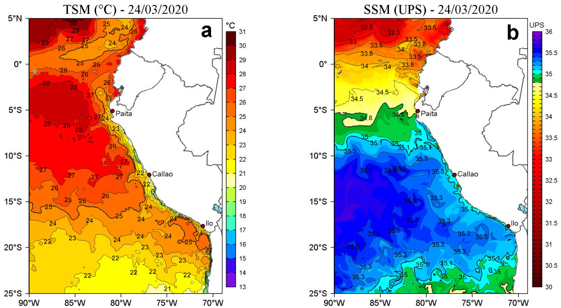
Figura 2. a) Temperatura superficial del mar (TSM, °C) y b) Salinidad superficial del mar (SSM, UPS), para el 24 de marzo de 2020. Datos: OSTIA-UKMO-L4-GLOB-v2.0 (UK Met Office, 2012; Donlon et al, 2012) disponible en https://podaac.jpl.nasa.gov/dataset/OSTIA-UKMO-L4-GLOB-v2.0 para (a) y Hybrid Coordinate Ocean Model v. GOF3 3.1 (HYCOM; Halliwell et al., 1998; 2000; Bleck, 2001) para (b). Procesamiento: LHF/AFIOF/DGIOCC/IMARPE.
