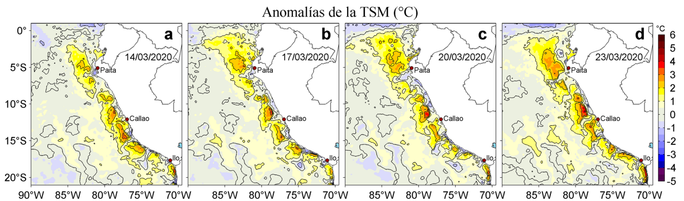
Figura 3. Anomalías de la temperatura superficial del mar (TSM, °C) para los días: a) 14, b) 17, c) 20 y d) 23 de marzo de 2020. Las anomalías se calcularon respecto de la climatología para el periodo 2007-2016. Datos: OSTIA-UKMO-L4-GLOB-v2.0 (UK Met Office, 2012; Donlon et al, 2012). Procesamiento: LHFM/AFIOF/DGIOCC/IMARPE.
