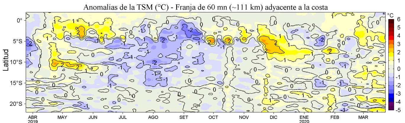
Figura 4. Variación promedio de las anomalías de la temperatura superficial del mar (TSM, °C) para una franja de 60 mn (~111 km) adyacente al litoral peruano para los últimos doce meses al 23 de marzo de 2020. Datos: OSTIA-UKMO-L4-GLOB-v2.0 (UK Met. Office, 2012; Donlon et al, 2012) disponible en https://podaac.jpl.nasa.gov/dataset/OSTIA-UKMO-L4-GLOB-v2.0 . Las anomalías se calcularon con respecto al periodo 2007-2016. Procesamiento: LHFM/AFIOF/DGIOCC/IMARPE.
