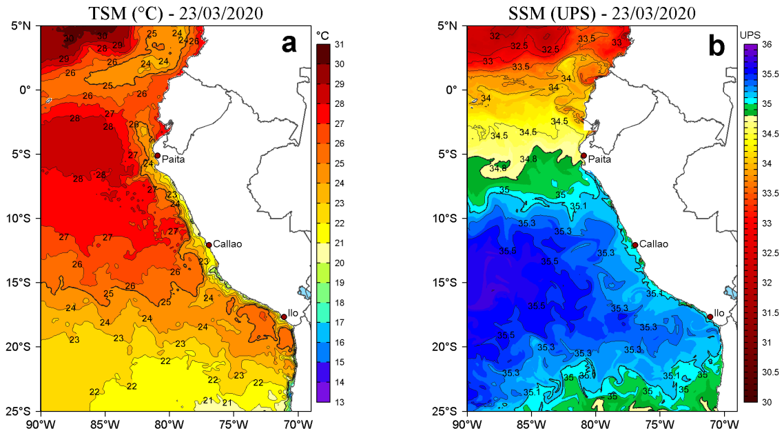
Figura 2. a) Temperatura superficial del mar (TSM, °C) y b) Salinidad superficial del mar (SSM, UPS), para el 23 de marzo de 2020. Datos: OSTIA-UKMO-L4-GLOB-v2.0 (UK Met Office, 2012; Donlon et al, 2012) disponible en https://podaac.jpl.nasa.gov/dataset/OSTIA-UKMO-L4-GLOB-v2.0 para (a) y Hybrid Coordinate Ocean Model v. GOFS 3.1 (HYCOM; Halliwell et al., 1998; 2000; Bleck, 2001) para (b). Procesamiento: LHFM/AFIOF/DGIOCC/IMARPE.
