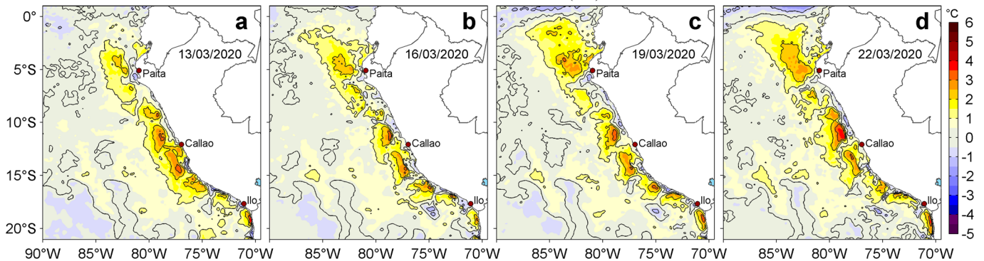
Figura 3. Anomalías de la temperatura superficial del mar (TSM, °C) para los días: a) 13, b) 16, c) 19 y d) 22 de marzo de 2020. Las anomalías se calcularon respecto de la climatología para el periodo 2007-2016. Datos: OSTIA-UKMO-L4-GLOB-v2.0 (UK Met Office, 2012; Donlon et al, 2012). Procesamiento: LHF/AFIOF/DGIOCC/IMARPE.
