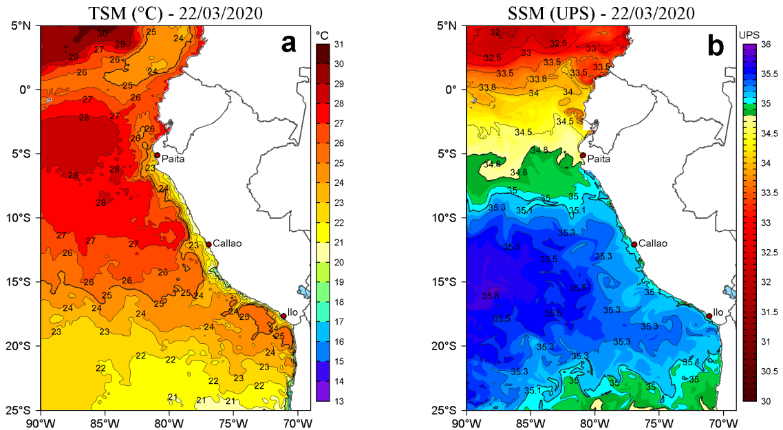
Figura 2. a) Temperatura superficial del mar (TSM, °C) y b) Salinidad superficial del mar (SSM, UPS), para el 22 de marzo de 2020. Datos: OSTIA-UKMO-L4-GLOB-v2.0 (UK Met Office, 2012; Donlon et al, 2012) disponible en https://podaac.jpl.nasa.gov/dataset/OSTIA-UKMO-L4-GLOB-v2.0 para (a) y Hybrid Coordinate Ocean Model v. GOFS 3.1 (HYCOM; Halliwell et al., 1998; 2000; Bleck, 2001) para (b). Procesamiento: LHF/AFIOF/DGIOCC/IMARPE.
